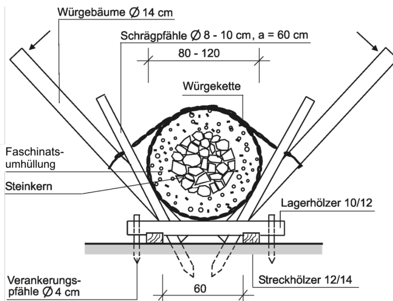
15-12 Senkfaschine (Querschnitt)
