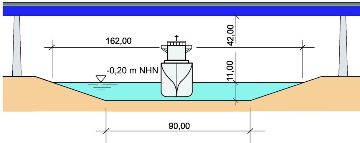
11-2 Querschnitt des Nord-Ostsee-Kanals
