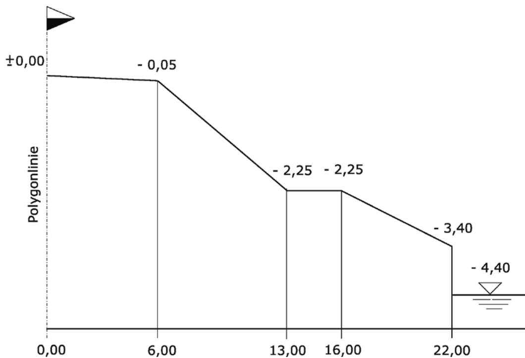
9-2 Uferanschlussprofil des linken Ufers bei km 65,4 (Handskizze)
