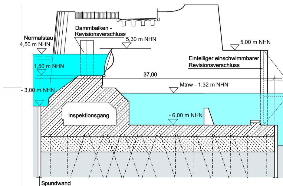
16-4 Klappenwehr in Bremen/Weser (Inbetriebnahme 1993)
