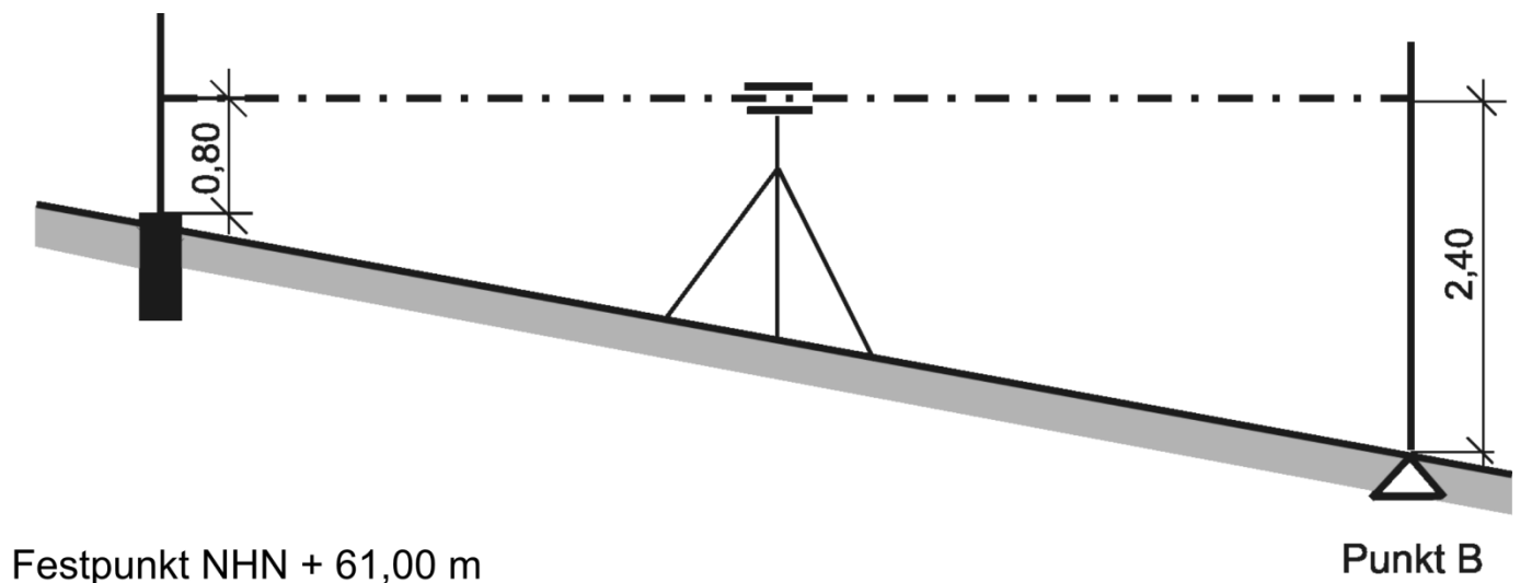
8-4 Messung des Höhenunterschieds zwischen zwei Punkten
