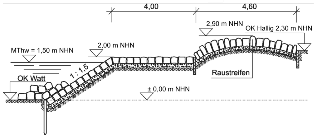
19-12 Deckwerk einer Hallig mit Raustreifen (Igel)
