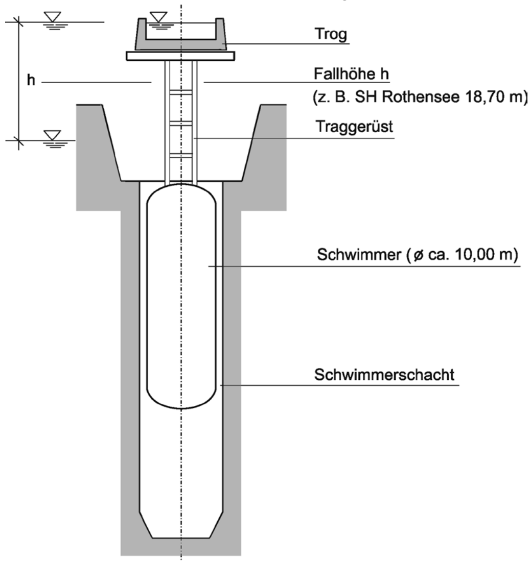
16-20 Schwimmerhebwerk (Querschnitt) - Schraubenspindeln zum Antrieb nicht dargestellt -
