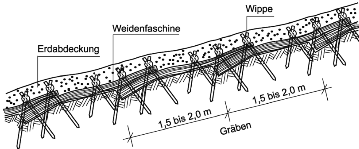
15-17 Spreutlage (Querschnitt durch die Böschung)
