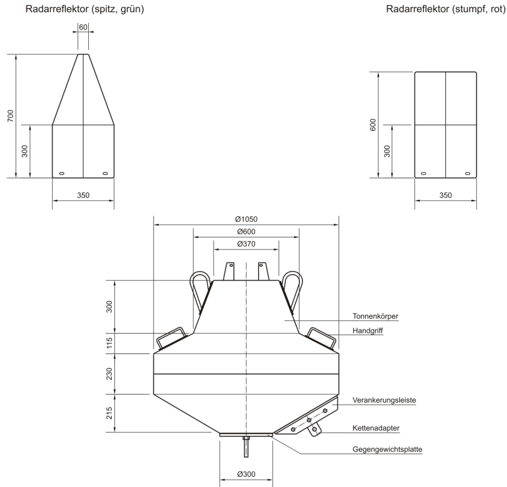
13-4 Binneneinheitstonne
