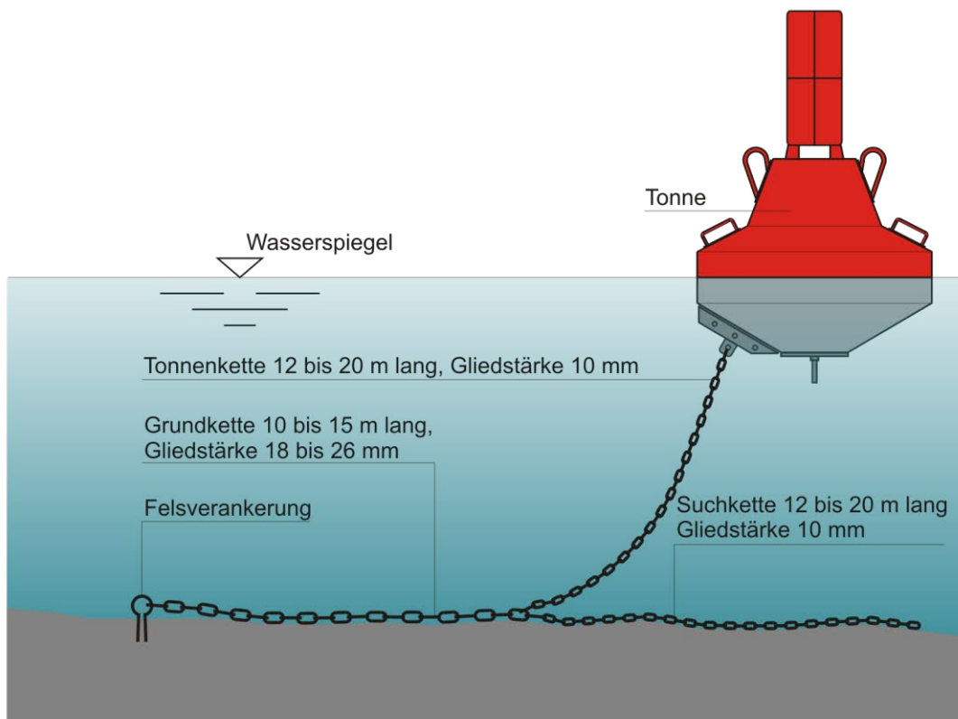
13-6 Tonneverankerung auf felsiger Flusssohle
