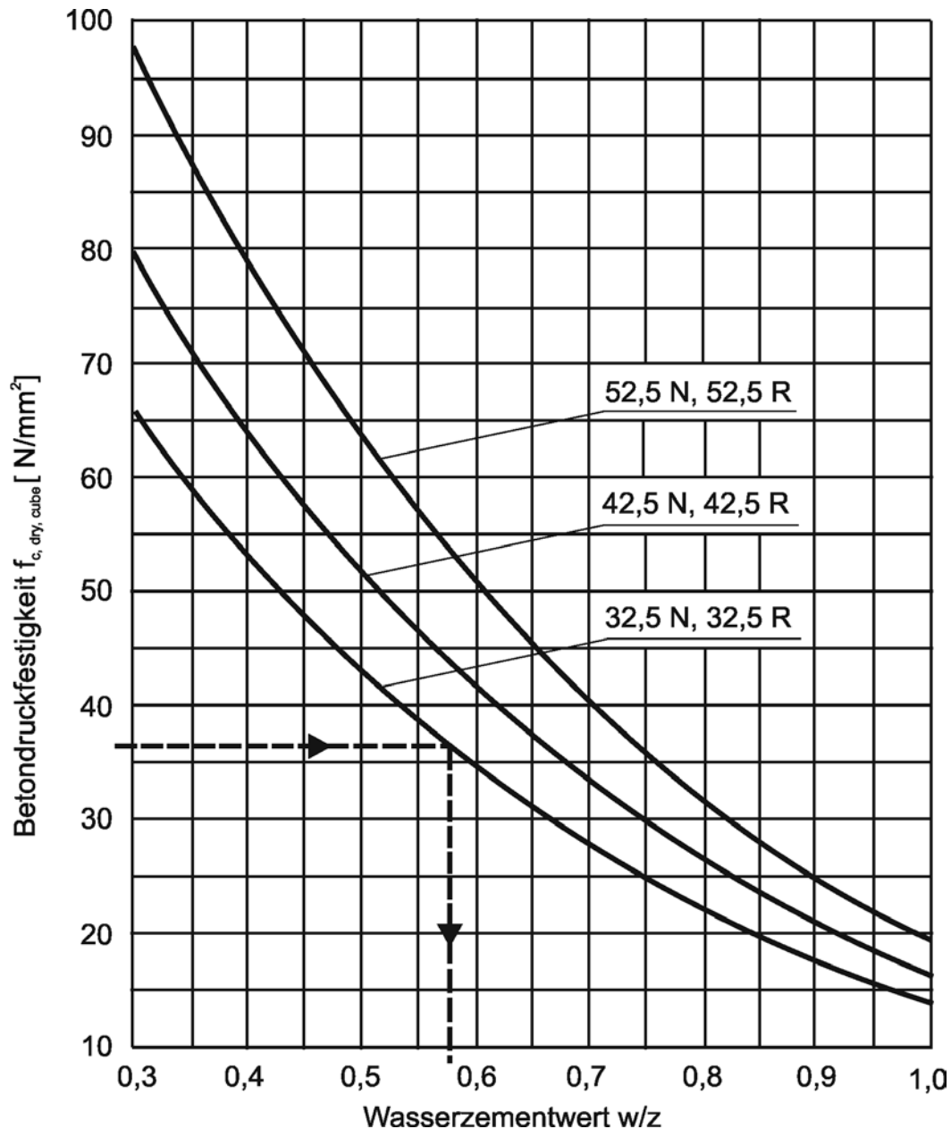
6-12 Zusammenhang zwischen Betondruckfestigkeit, Festigkeitsklasse des Zements und Wasserzementwert (Walz-Diagramm)
