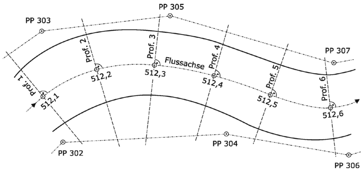
9-1 Festlegung des Profils
