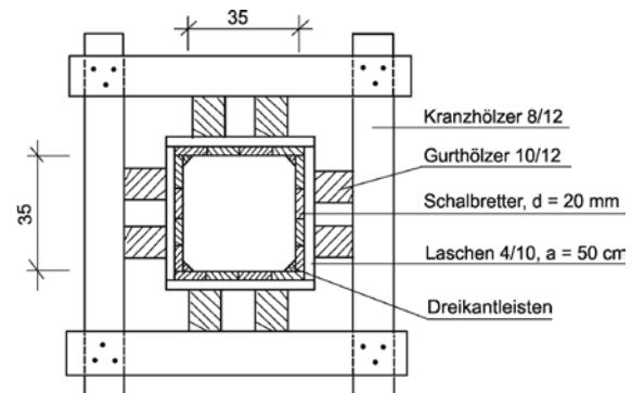
6-20 Schalung für eine Stahlbetonstütze (Querschnitt)
