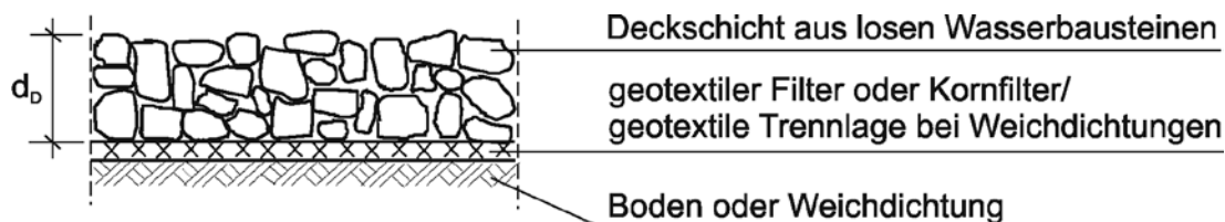
15-21 Durchlässige Deckschicht aus losen Wasserbausteinen (Schematische Darstellung im Querschnitt)
