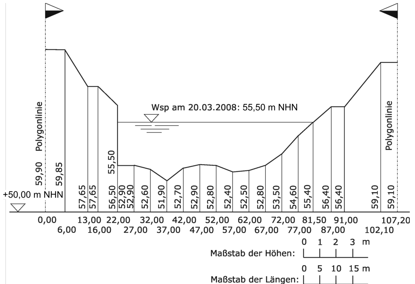
9-3 Querprofil bei Fluss-km 65,4
