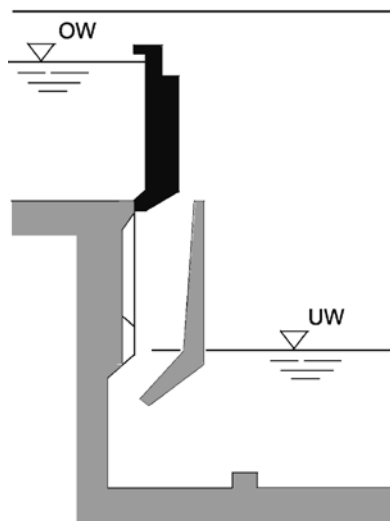
Senktor
