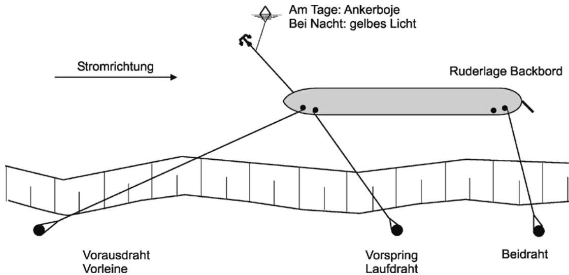
20-3 Festmachen eines Schiffes im Strom
