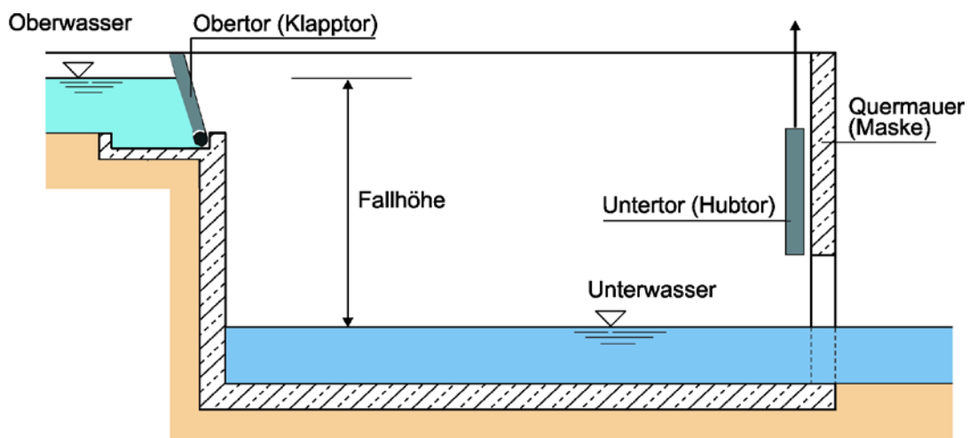
16-12 Schematischer Längsschnitt durch eine Schachtschleuse
