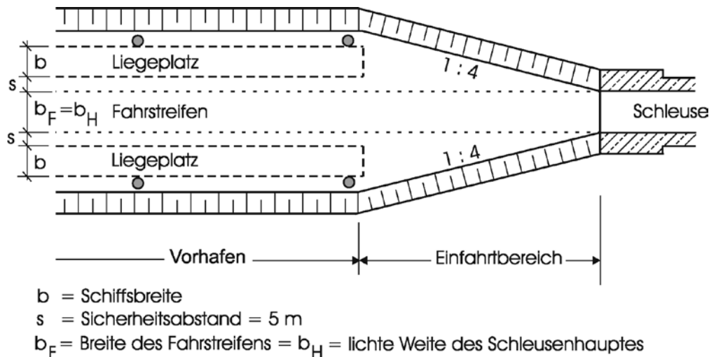
16-18 Schleusenvorhafen
