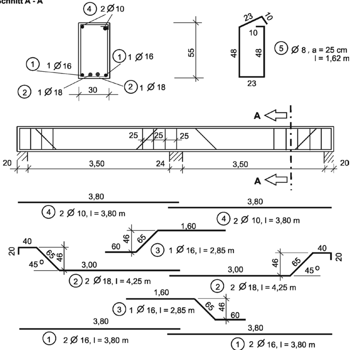
6-25 Bewehrung eines Betonbalkens
