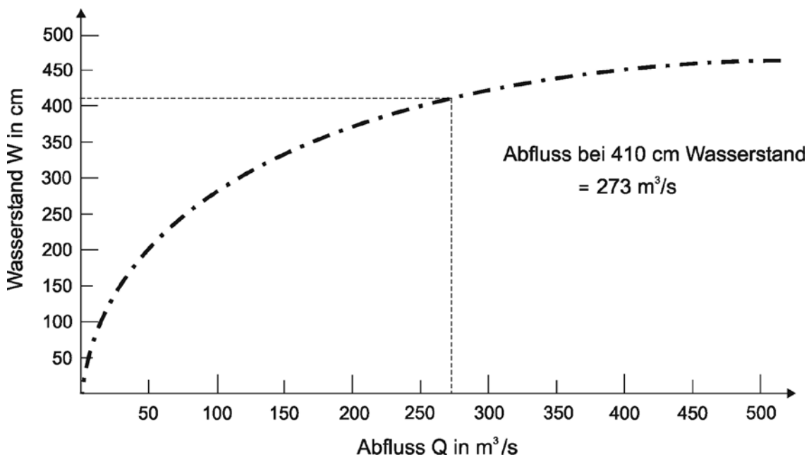
10-15 Abflusskurve
