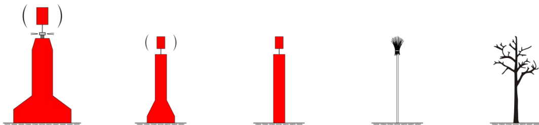
13-56 Backbordseite des Fahrwassers
