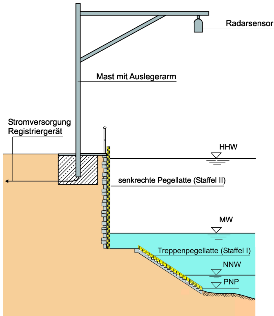
10-11 Radarpegel
