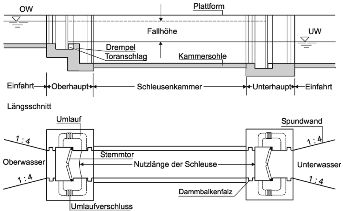
16-11 Längsschnitt und Draufsicht einer Schleuse
