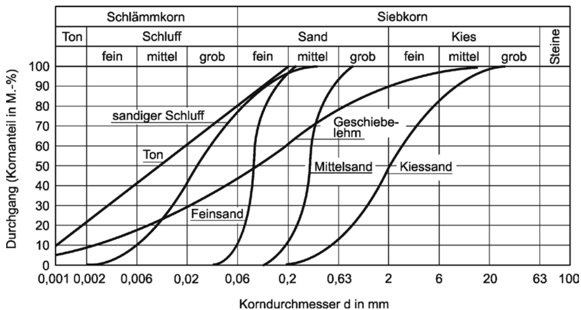
6-31 Kornverteilungslinien
