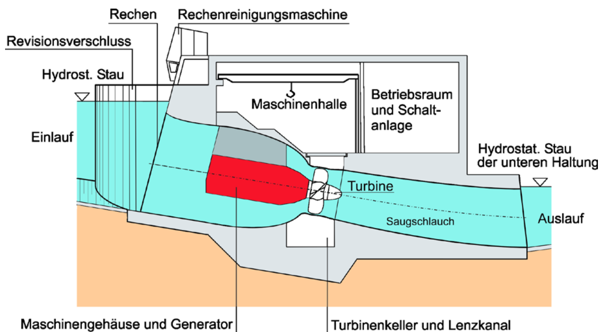
16-30 Querschnitt eines Kraftwerkes mit Kaplan-Rohrturbine
