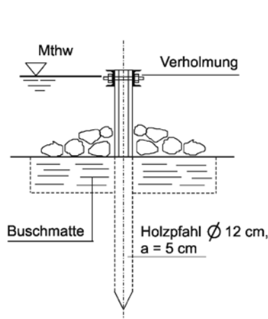
19-13 Einreihige Pfahlbuhne (Querschnitt)
