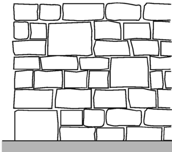
Unregelmäßiges Schichtenmauerwerk
