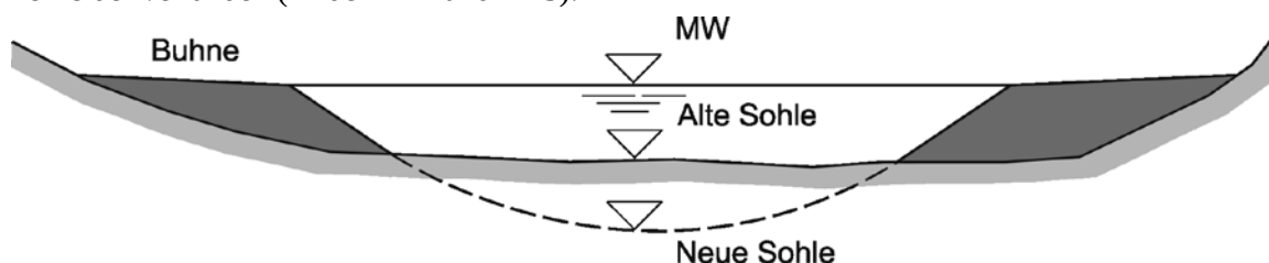
12-4 Wirkung der Mittelwasserregelung durch Buhnen
