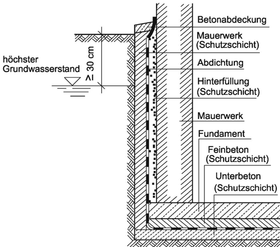
6-29 Außenhautabdichtung
