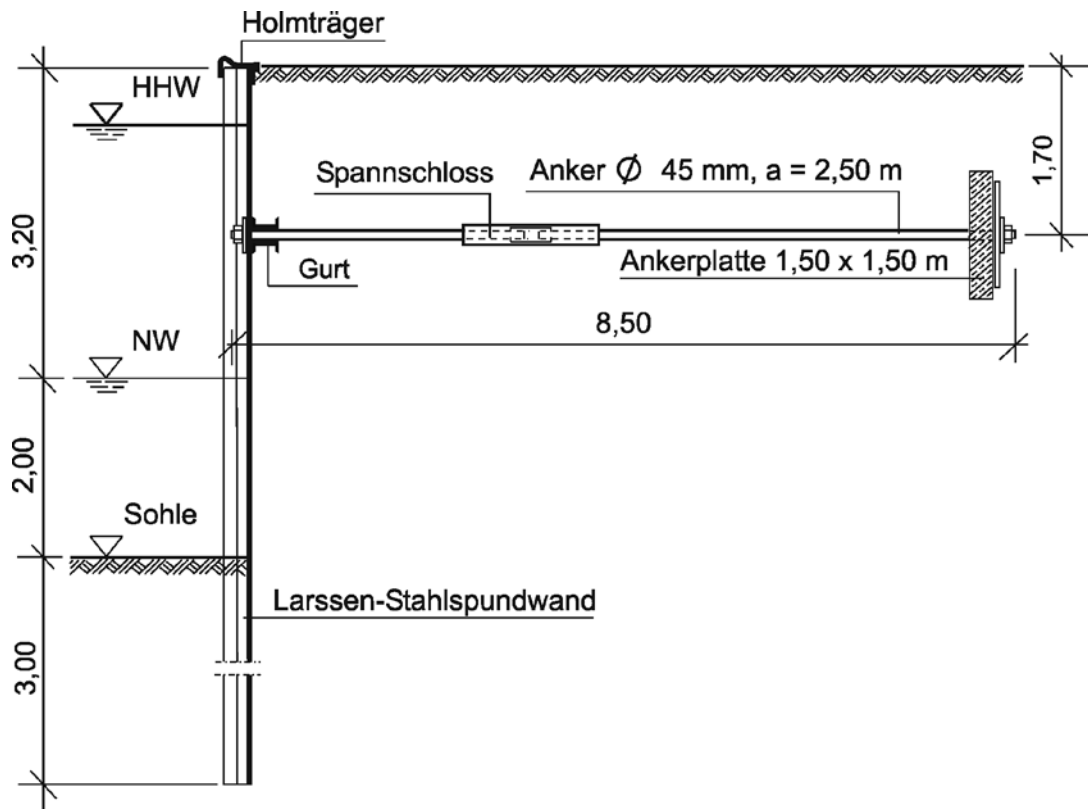
15-32 Stahlspundwand mit Rückverankerung
