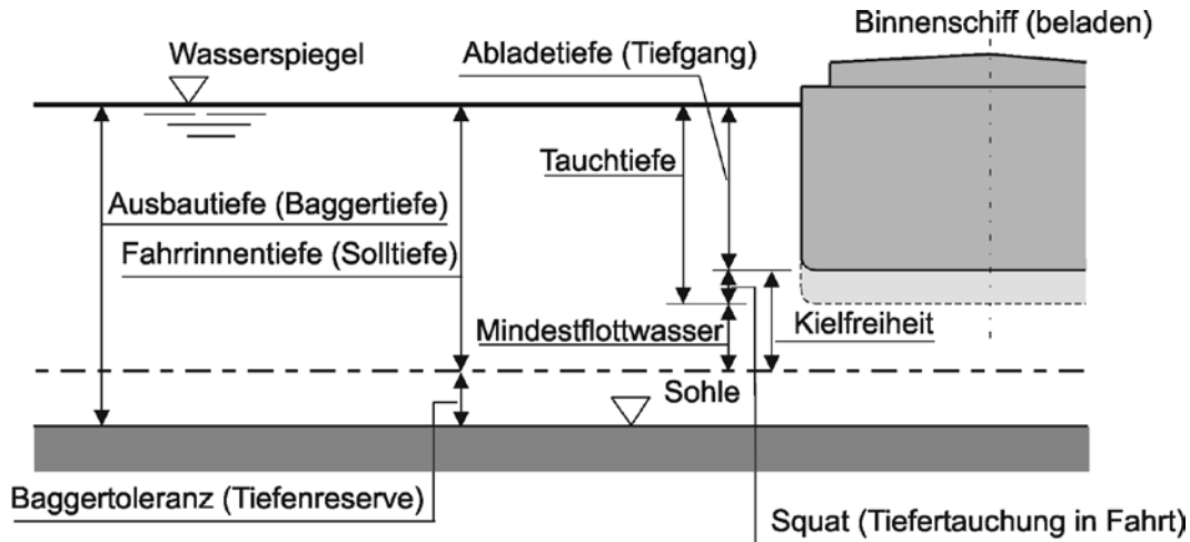
13-1 Schiff und Fahrrinne
