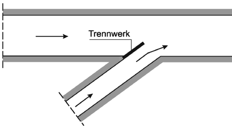
12-8 Trennwerk
