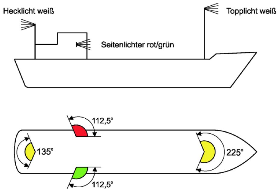
21-1 Lichterführung eines Maschinenfahrzeuges bis 110 m in Fahrt
