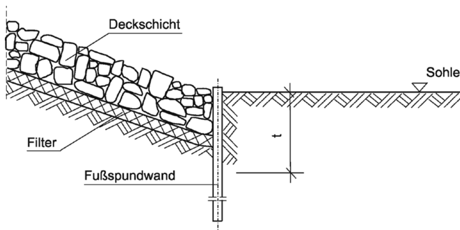
15-30 Fußspundwand
