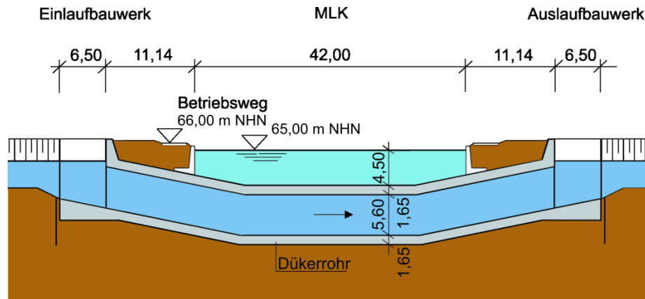
16-29 Längsschnitt eines Dükers unter dem Mittellandkanal
