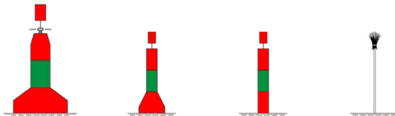
13-58 Backbordseite - Abzweigung/Einmündung
