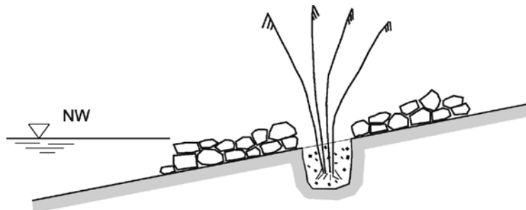
15-2 Ballenpflanzung
