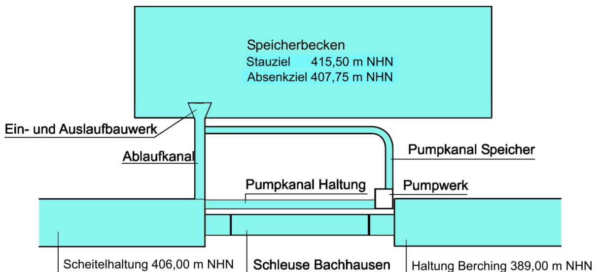
17-2 Draufsicht des Dürrho-Speichers am Main-Donau-Kanal (Schematische Darstellung)
