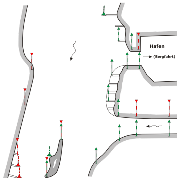
13-18 Zusammenspiel der Bilder 13-13 bis 13-17
