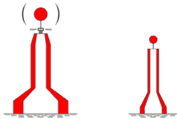
13-54 Bezeichnung der Zufahrt zu Fahrwassern und der Mitte von Schifffahrtswegen
