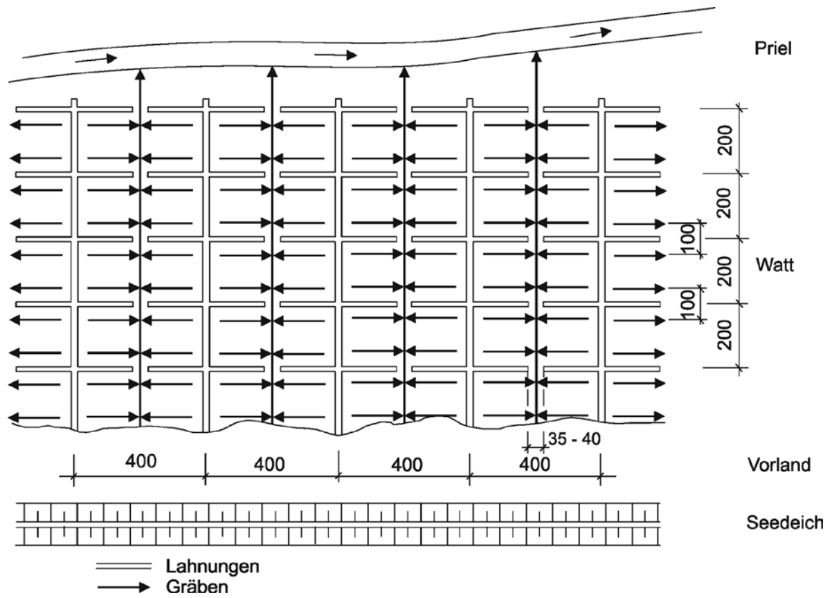
19-16 Lahnungssystem
