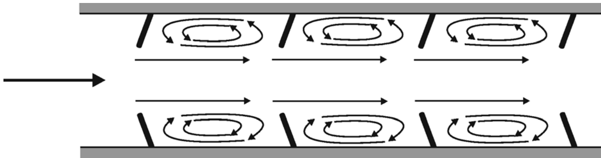
12-5 Funktionsweise inklinanter Buhnen
