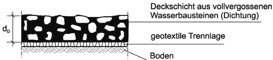
15-25 Dichte Deckschicht aus vollvergossenen Wasserbausteinen (Schematische Darstellung im Querschnitt)
