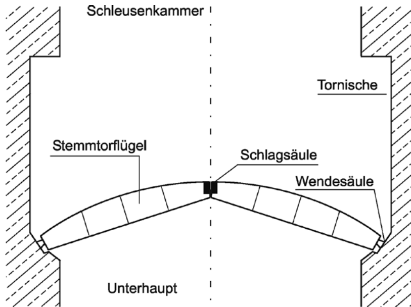
16-16 Stemmtor (Draufsicht)
