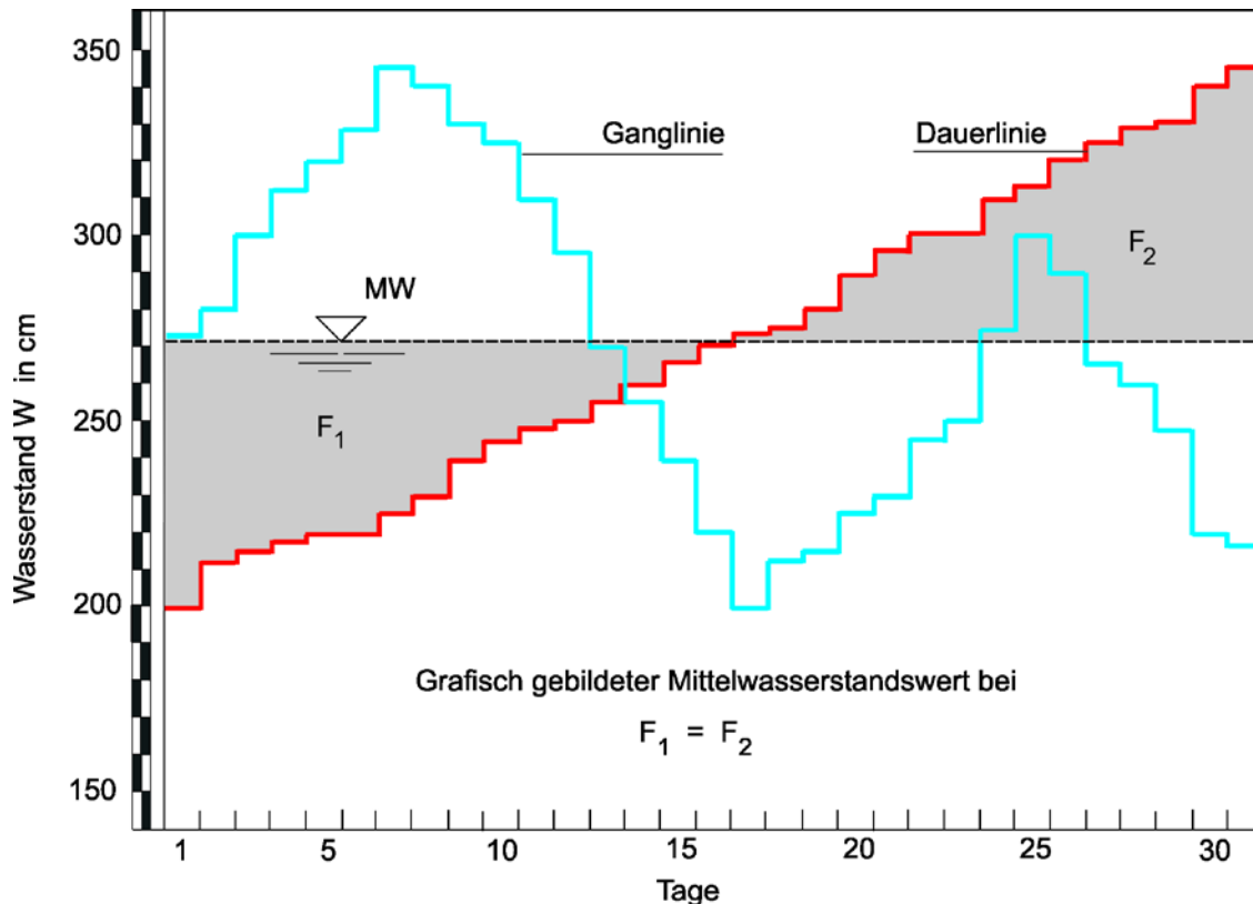
10-13 Wasserstands-Ganglinie und Wasserstands-Dauerlinie eines Monats
