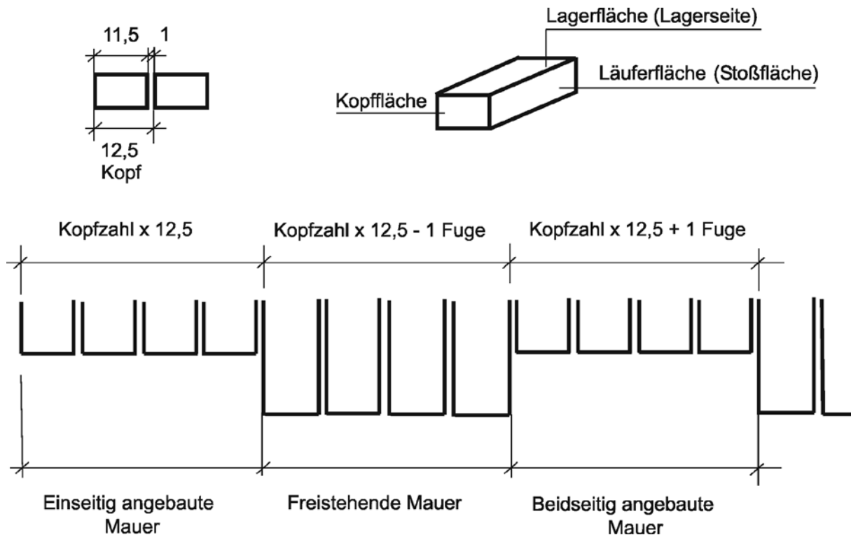
6-7 Schema für die Berechnung der Mauerlängen
