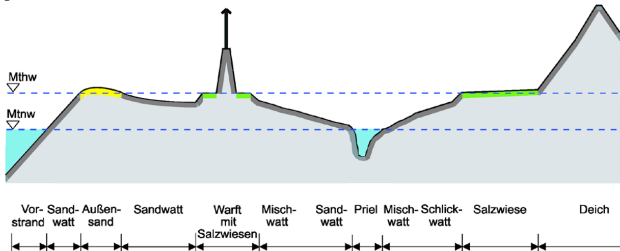
19-2 Schematischer Querschnitt des Wattenmeeres in Nordfriesland (überhöhte Darstellung) (Landesbetrieb für Küstenschutz, Nationalpark und Meeresschutz Schleswig-Holstein – LKN-SH)
