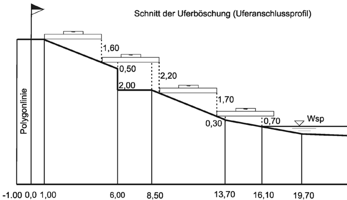
8-7 Handriss zu einer Staffelmessung
