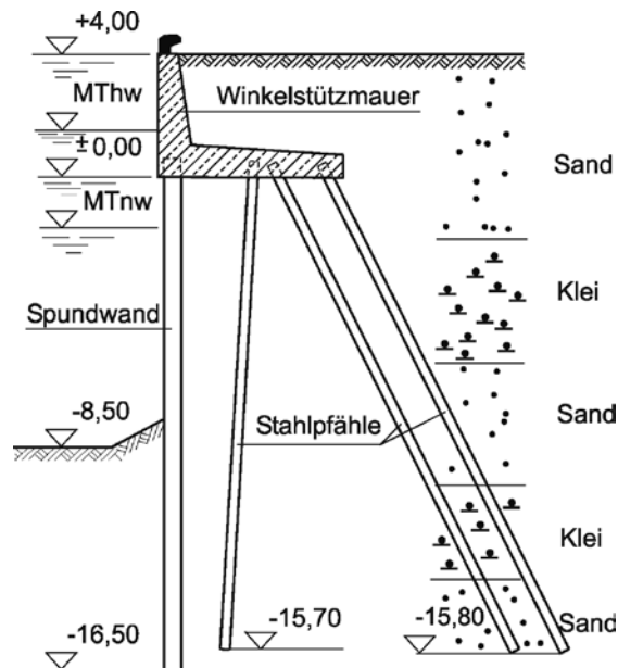
15-40 Pfahlrostbauwerk
