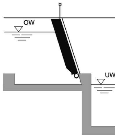
Klapptor
