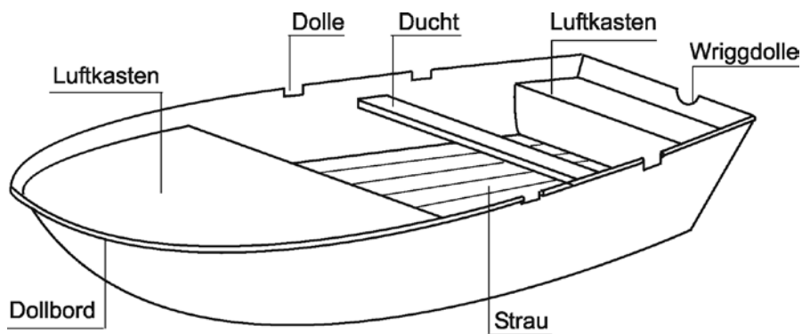
20-4 Bezeichnung der Einzelteile eines Nachens
