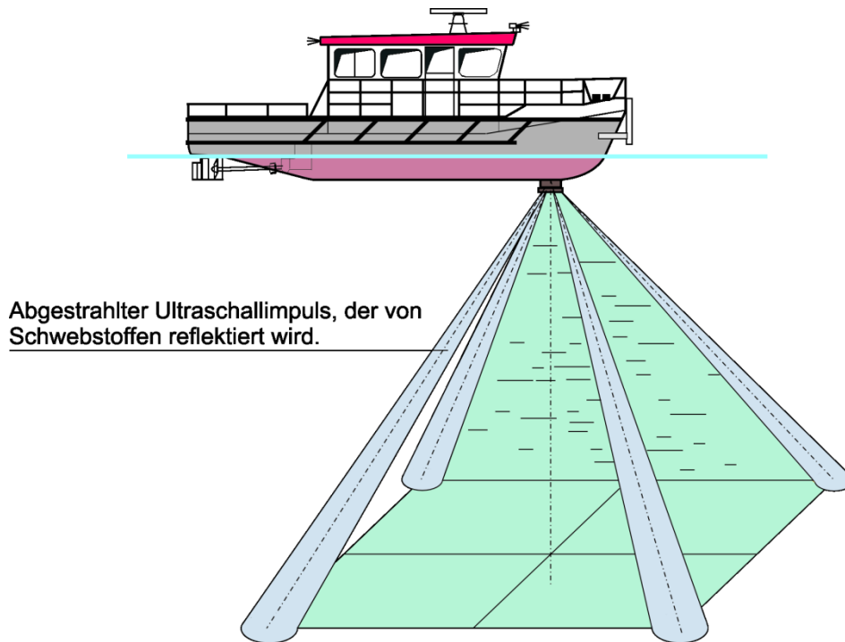
10-21 ADCP-Messprinzip
