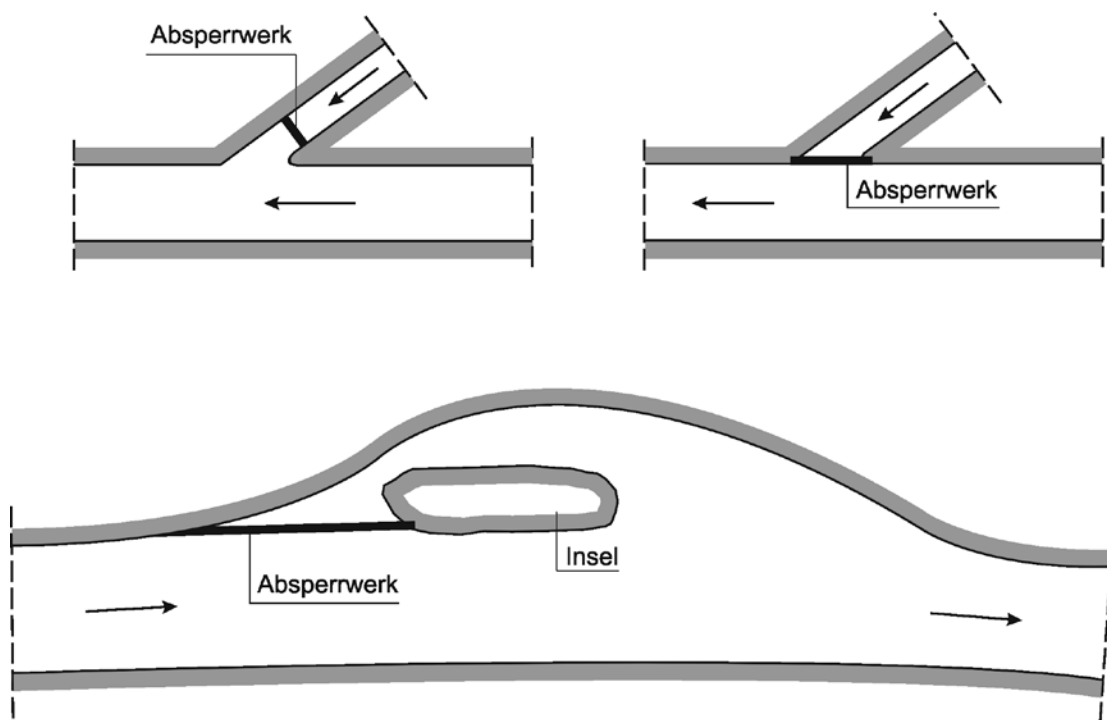
12-11 Absperrwerke
