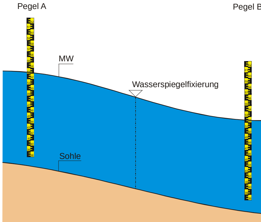
10-12 Wasserspiegelfixierung bei Mittelwasser (überhöhte Darstellung)
