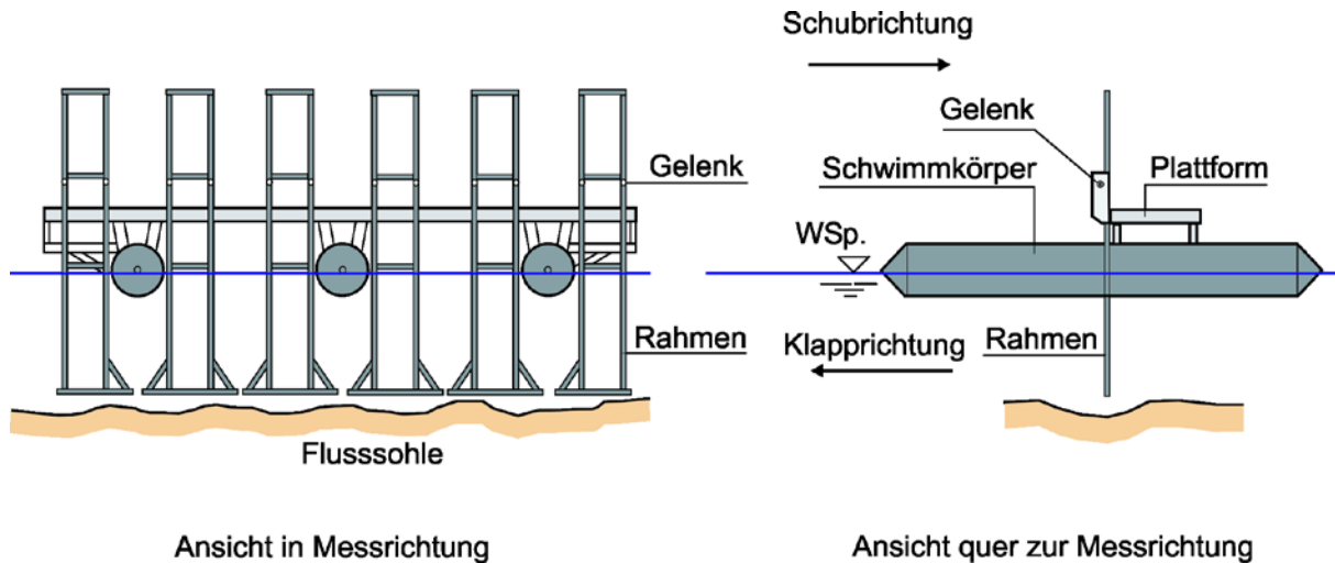
14-2 Mechanischer Peilrahmen (schematische Darstellung)
