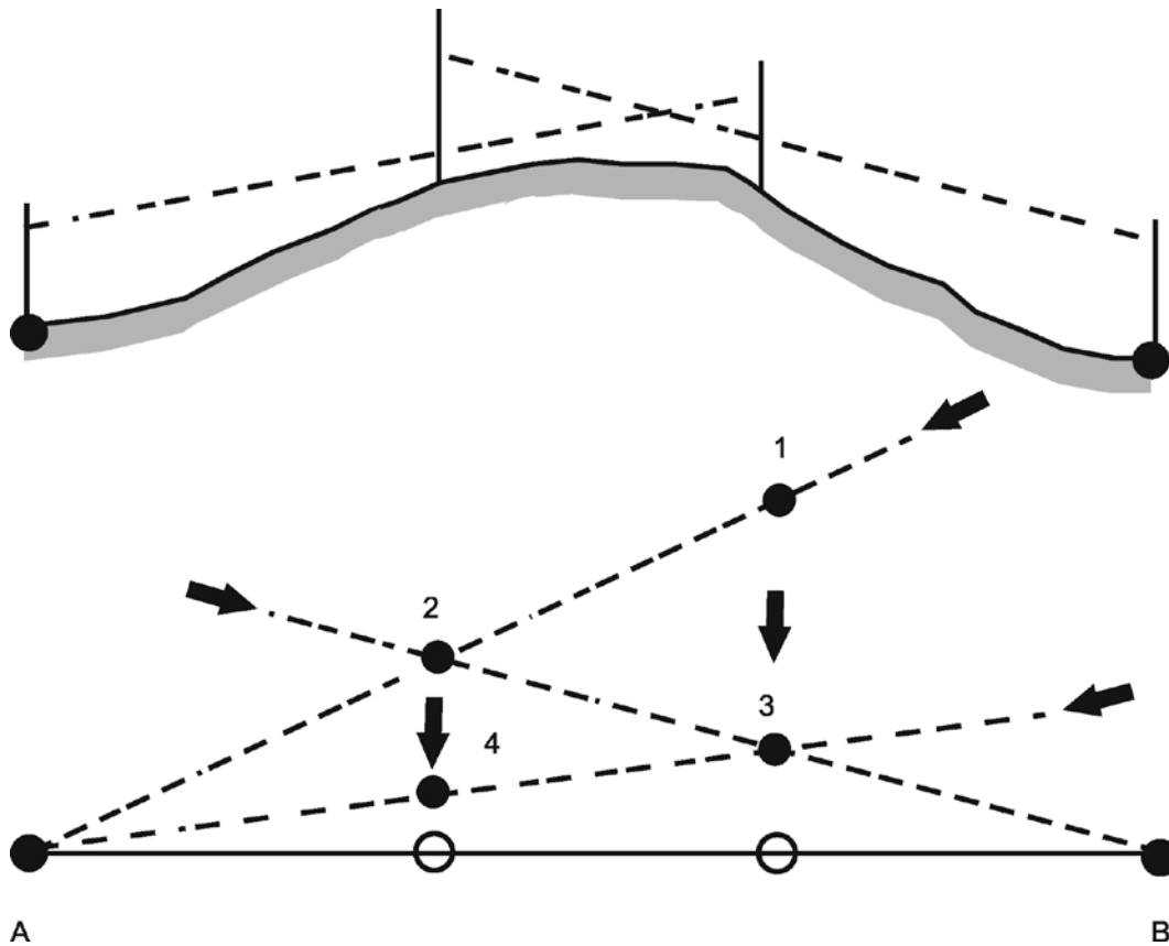
8-2 Einfluchten bei Gelände Hindernissen
