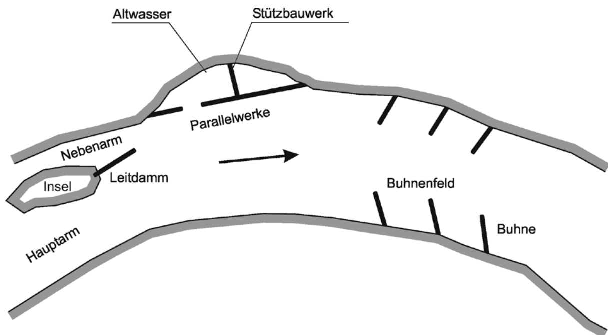
12-3 Bauwerke der Mittelwasserregelung
