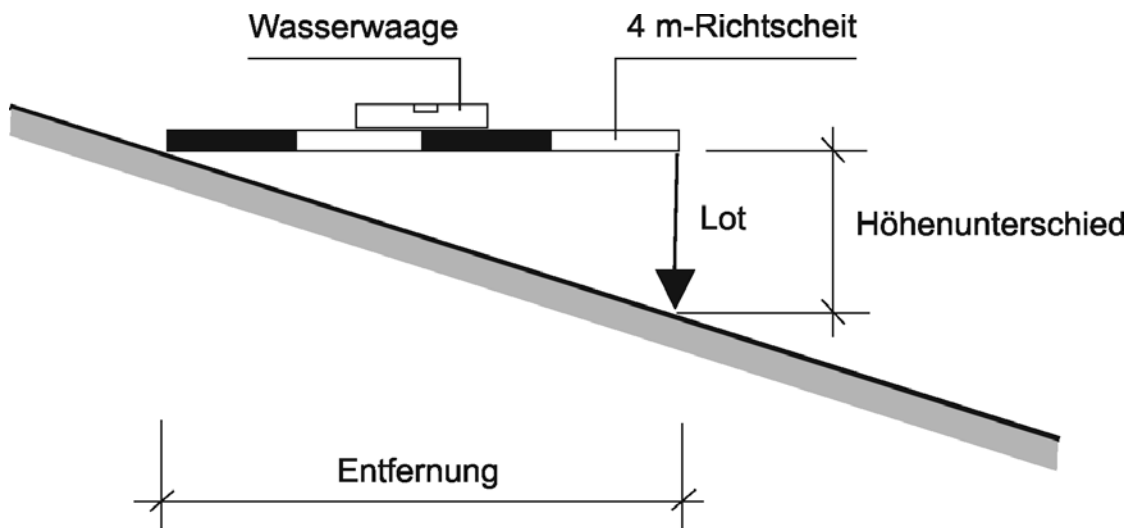
8-6 Staffelmessung
