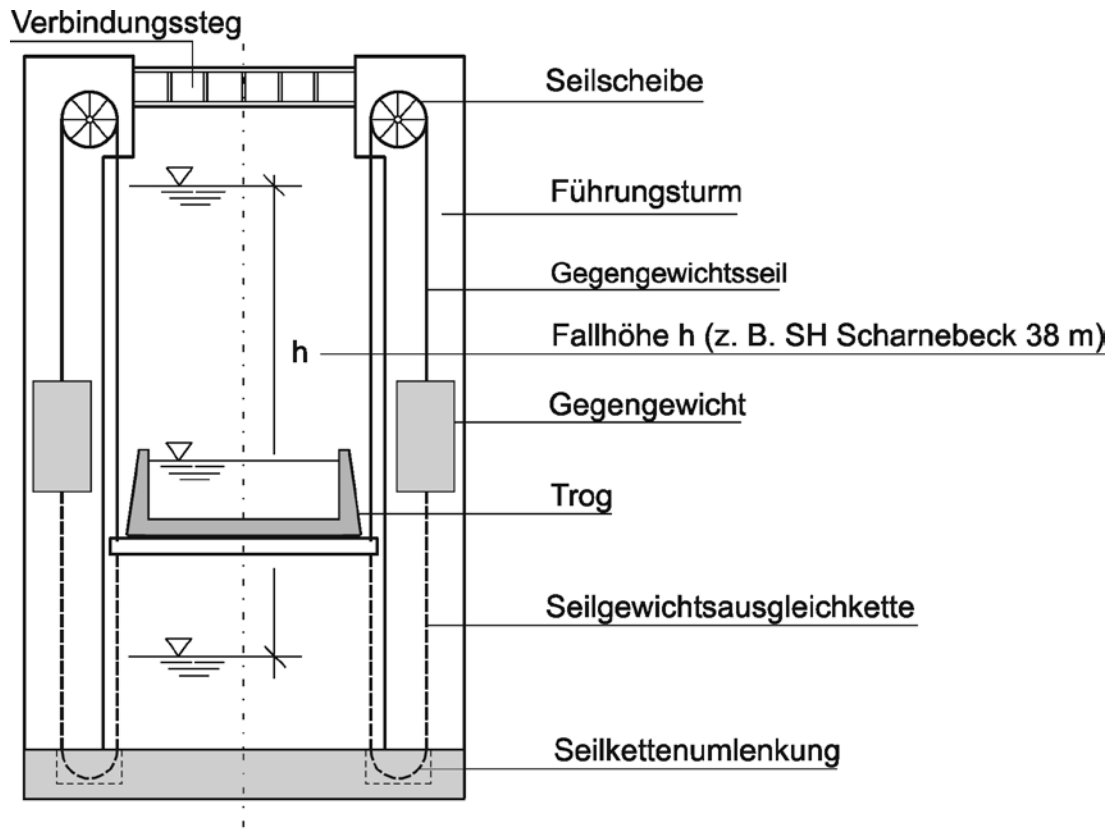
16-21 Gegengewichtshebwerk (Querschnitt) - Antriebs Elemente (Spindeln, Zahnstangen) nicht dargestellt -
