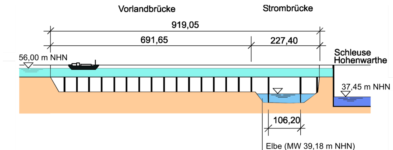
16-23 Längsschnitt der Kanalbrücke Magdeburg (überhöhte Darstellung)
