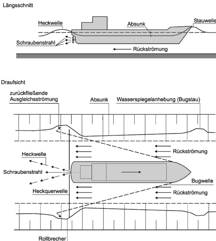
13-3 Hydraulische Belastung einer Böschung durch das fahrende Schiff
