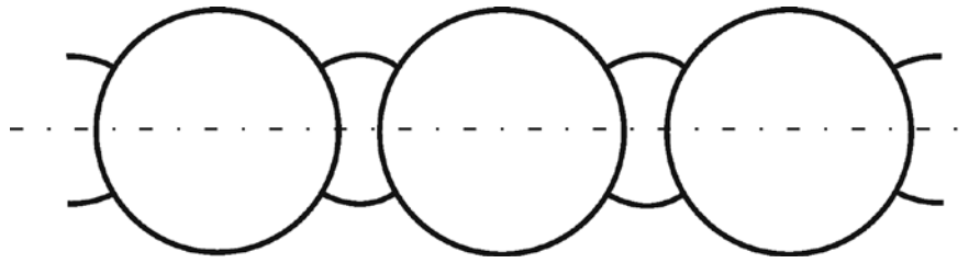
15-33 Schema (Draufsicht) eines Kreiszellenfangedammes
