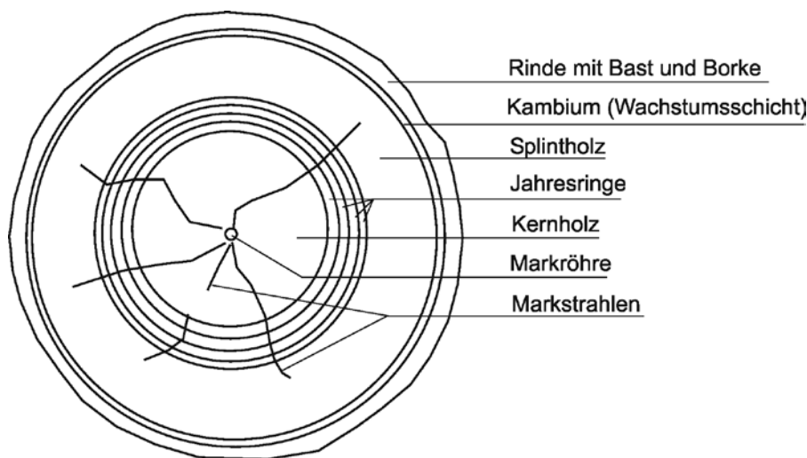
6-34 Aufbau des Holzes (Querschnitt)
