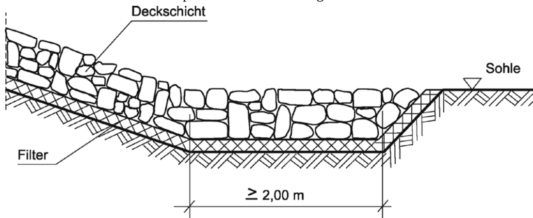
15-29 Fußvorlage
