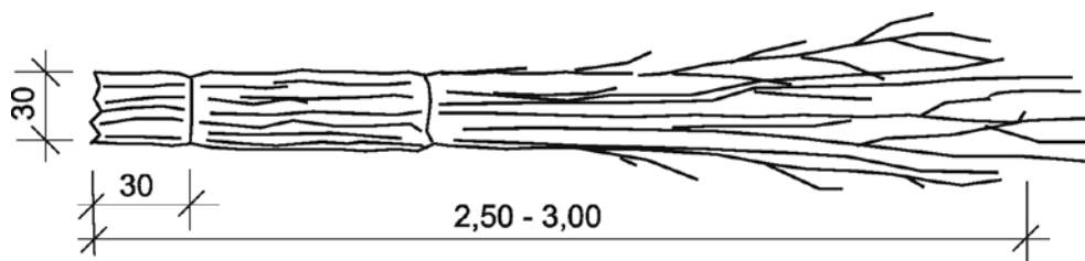
15-9 Faschine
