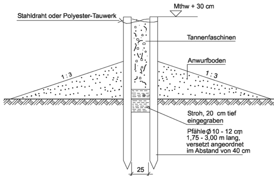
19-15 Lahnung (Querschnitt)
