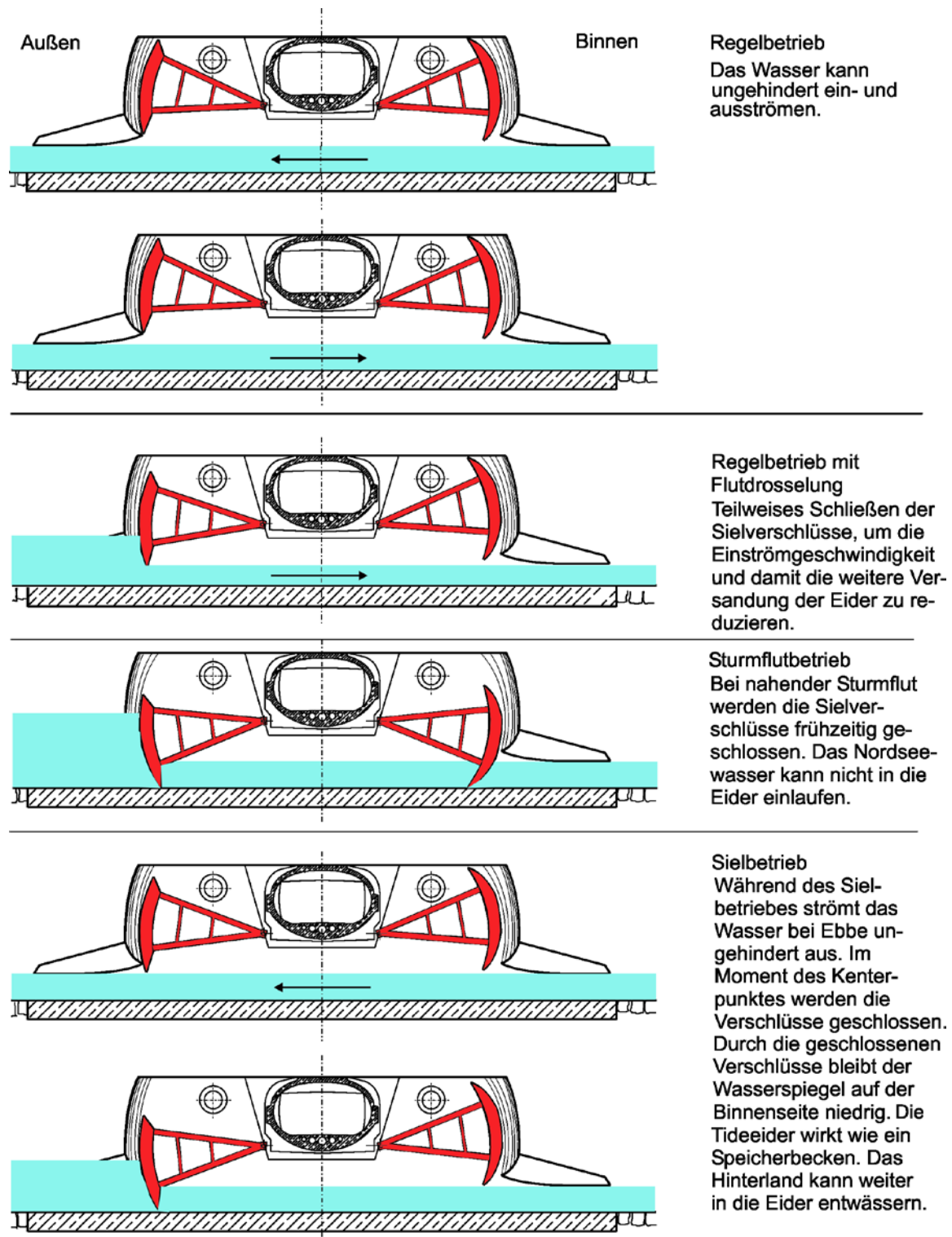
19-7 Betriebsformen des Eidersperrwerkes
