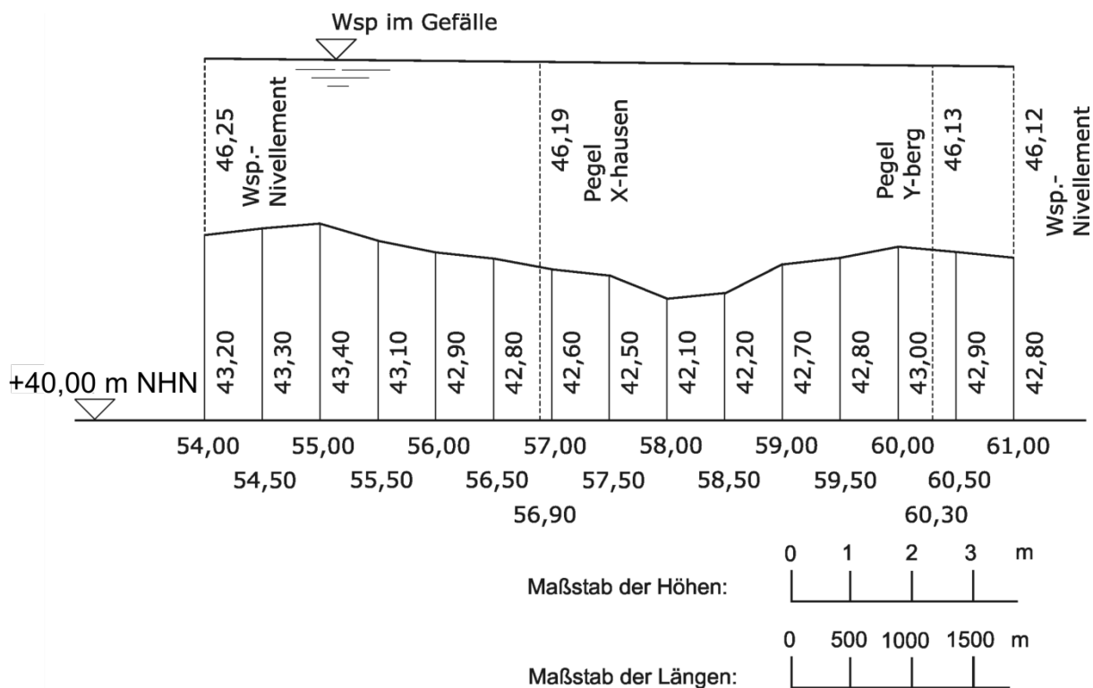
9-5 Längsprofil
