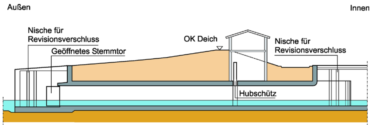
19-9 Längsschnitt eines Sieles
