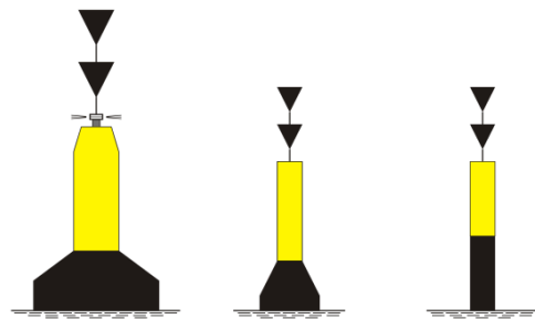
13-65 Süd-Kardinalzeichen
