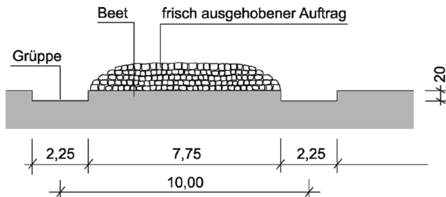
19-18 Querschnitt durch ein Gruppenfeld
