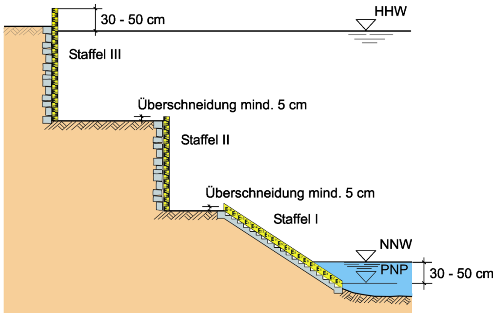
10-8 Pegelstaffel
