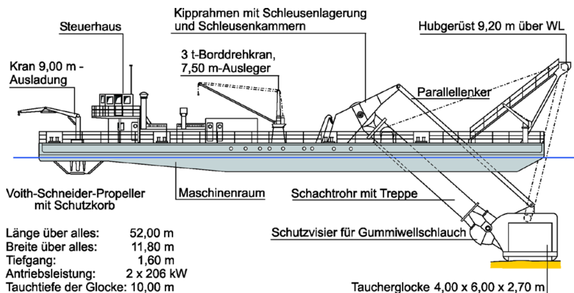
14-6 Taucherglockenschiff „Carl Straat“
