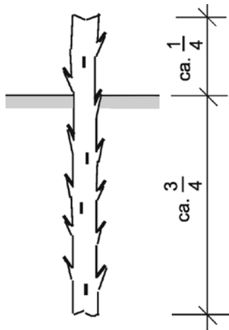
Setzstangenabmessungen: Durchmesser: 3 - 8 cm Länge: 100 - 250 cm
