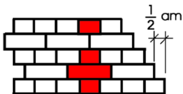
Kreuzverband
