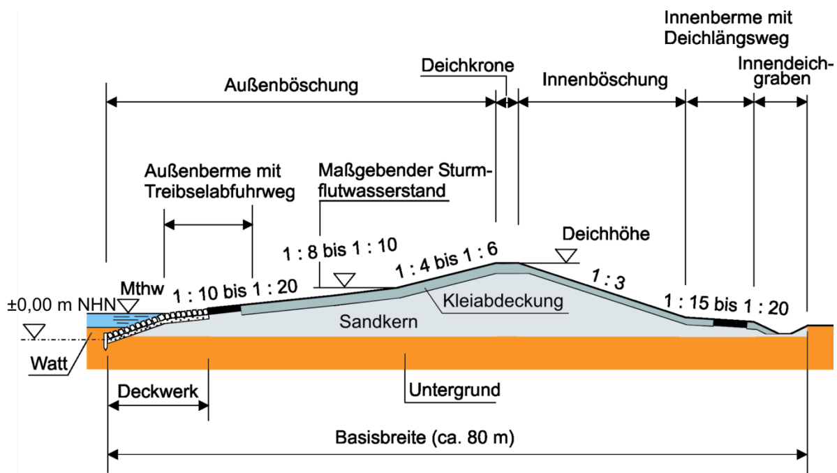
19-5 Schematischer Querschnitt eines Schardeiches (LKN-SH)
