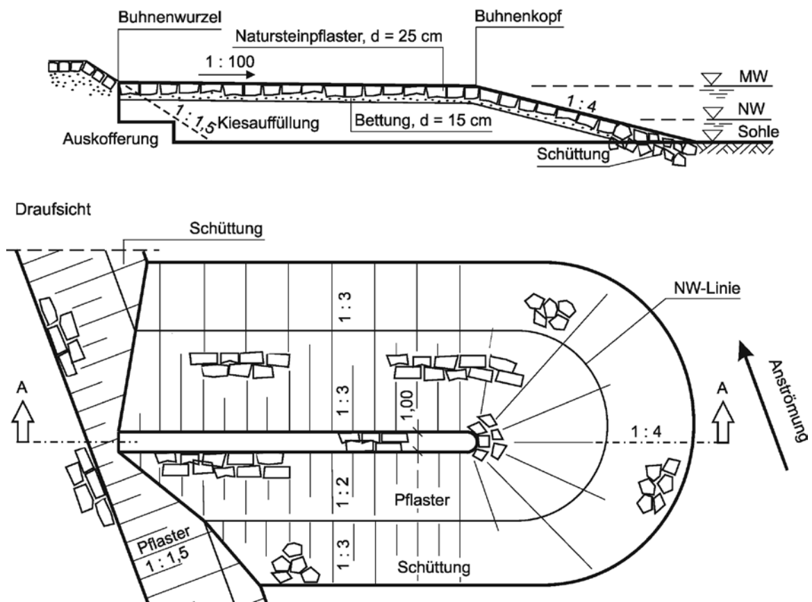
12-6 inklinante Steinbühne
