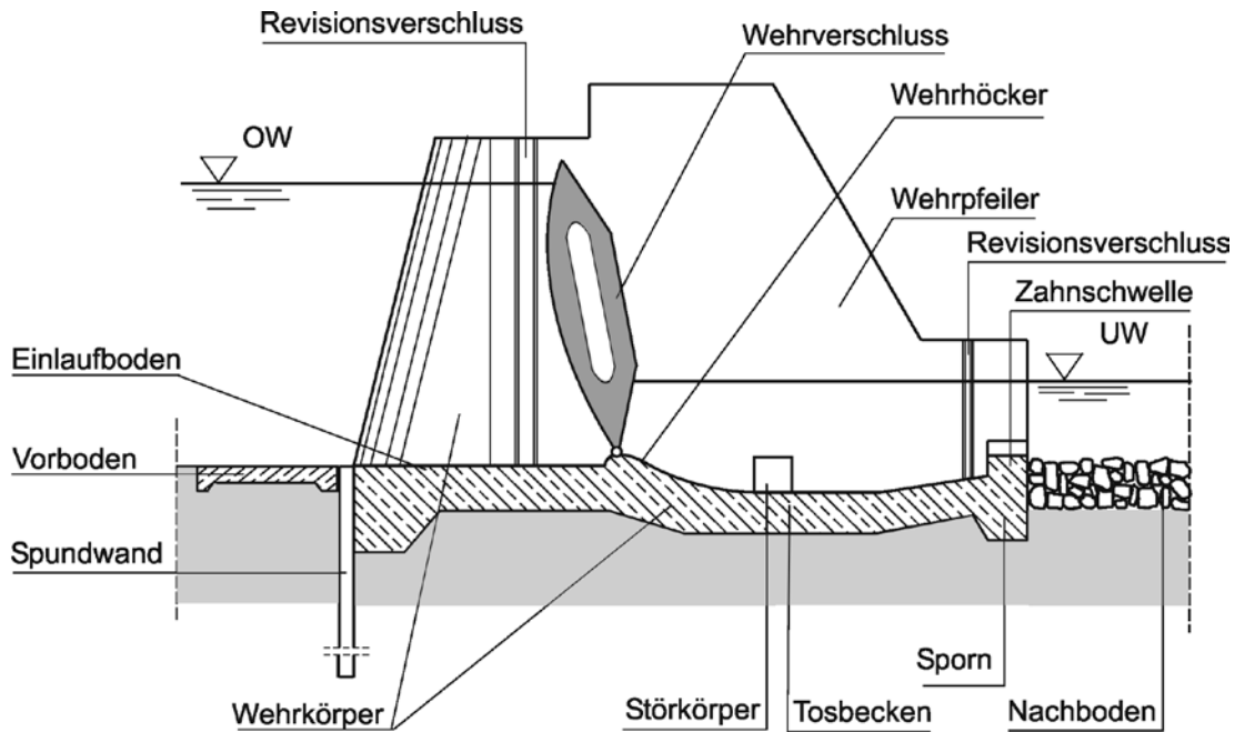
16-2 Bestandteile des beweglichen Wehres
