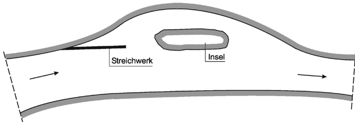
12-10 Streichwerk
