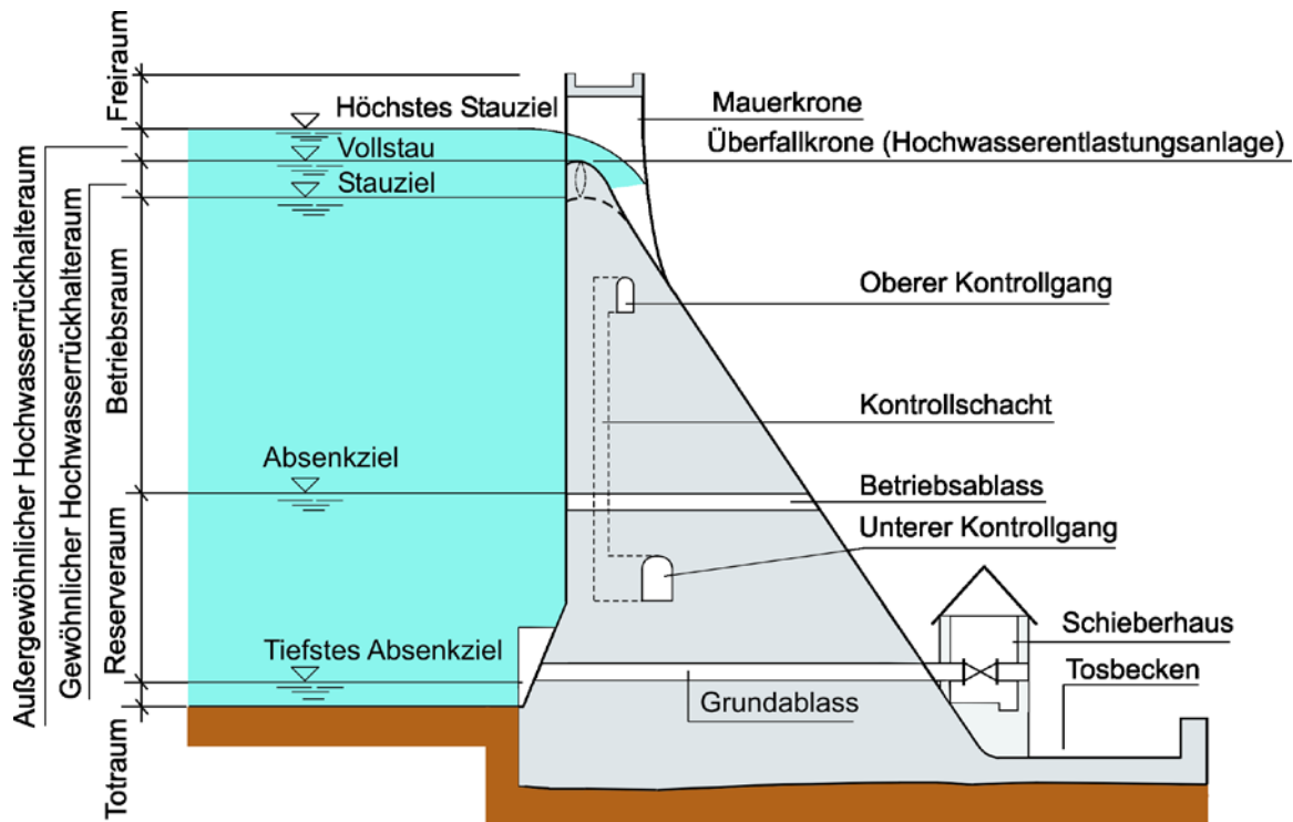
17-1 Speicherräume und Stauziele einer Talsperre
