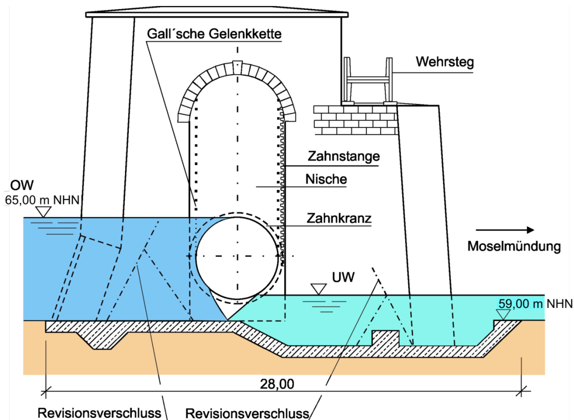
16-8 Walzenwehr der untersten Staustufe der Mosel in Koblenz (Inbetriebnahme 1951)
