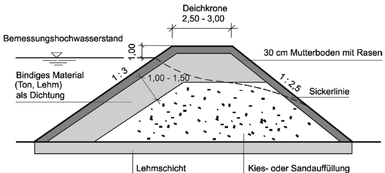
12-2 Querschnitt eines Deiches (überhöhte Darstellung)
