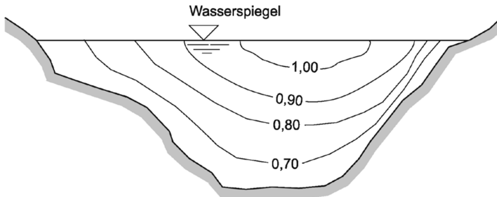
10-14 Geschwindigkeitsverteilung im Flussquerschnitt (Geschwindigkeit in m/s)
