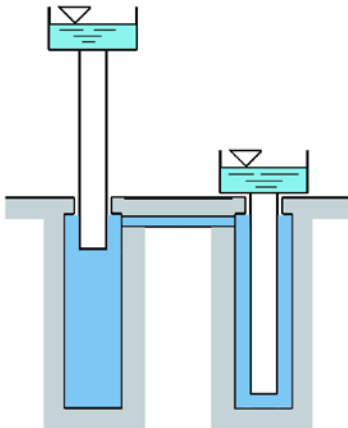
Presskolbenhebewerk
