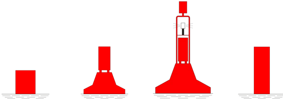
13-7 Rechte Seite - Fahrrinne
