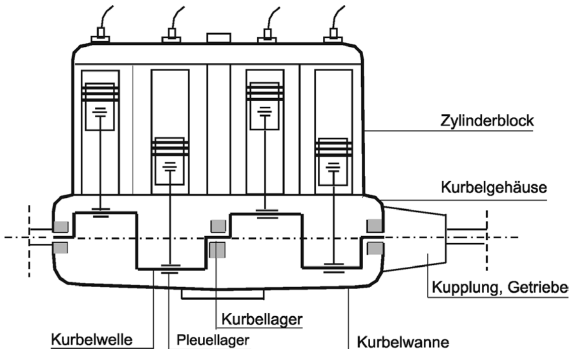
7-2 Otto-Viertaktmotor
