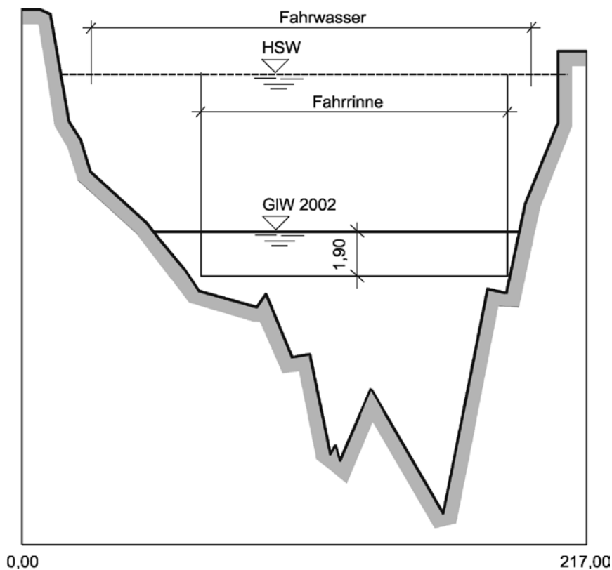
13-2 Fahrrinne und Fahrwasser (Querprofil bei Rhein-km 553,400 (Überhöhte Darstellung))
