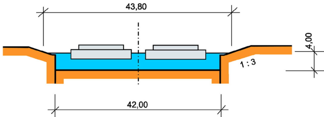
11-1 Regelquerschnitte für den Ausbau von Schifffahrtskanälen der Wasserstraßenklasse V
