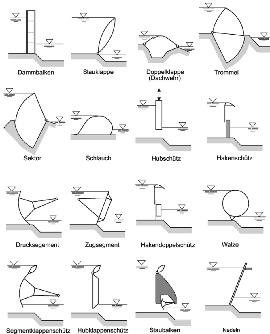
16-3 Funktionsweisen von Wehrverschlüssen
