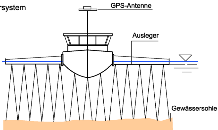
Fächerecholot
