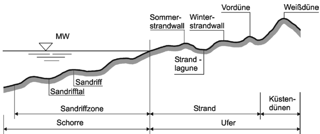
19-4 Schematischer Querschnitt einer Flachküste
