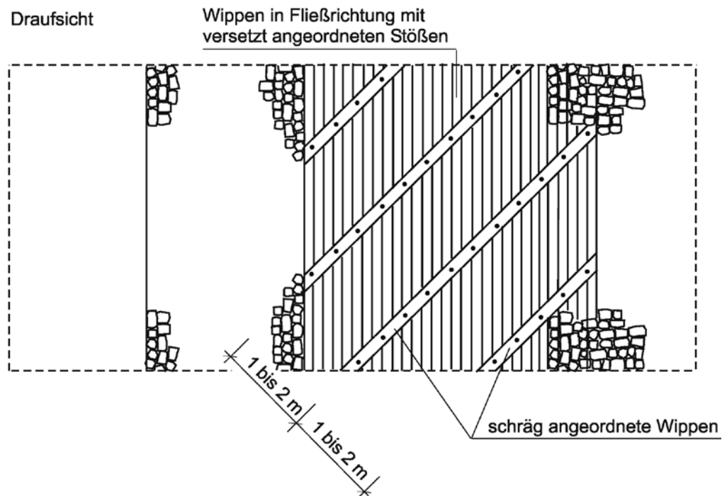
15-15 Faschinenmatte
