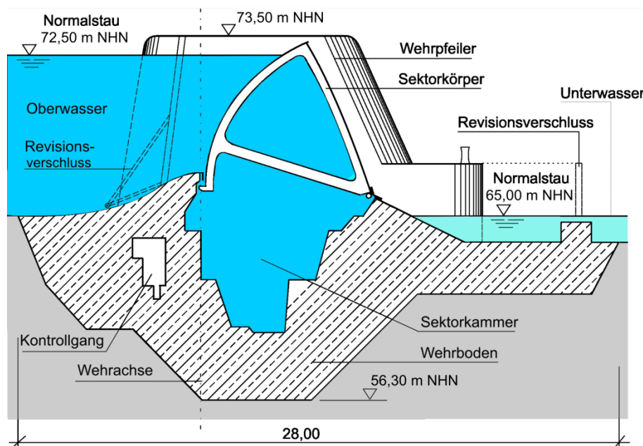
16-5 Sektorwehr Lehen/Mosel (Inbetriebnahme 1965)
