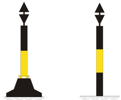
13-37 Ost-Kardinalzeichen
