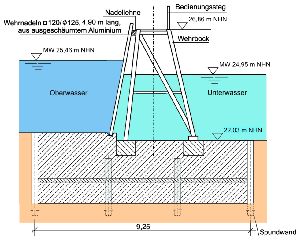
16-9 Nadelwehr Grätz/Untere Havel-Wasserstraße (Inbetriebnahme 2003; Ersatz eines Nadelwehres, Baujahr 1910)
