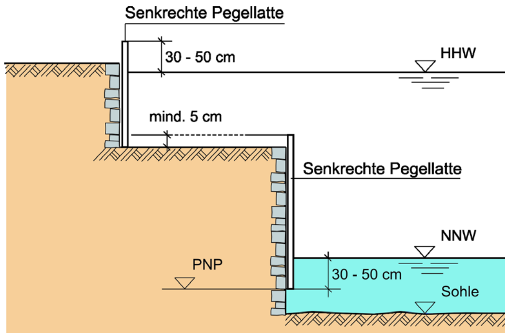
10-3 Lage des Pegelnulldpunktes
