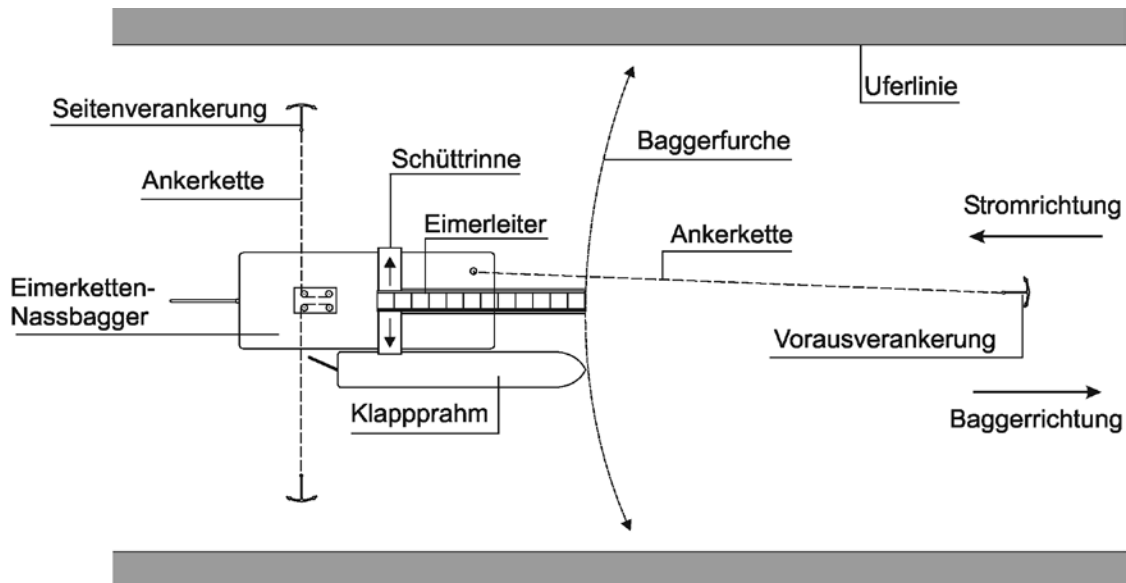
14-4 Arbeitsweise des Eimerketten-Nassbaggers
