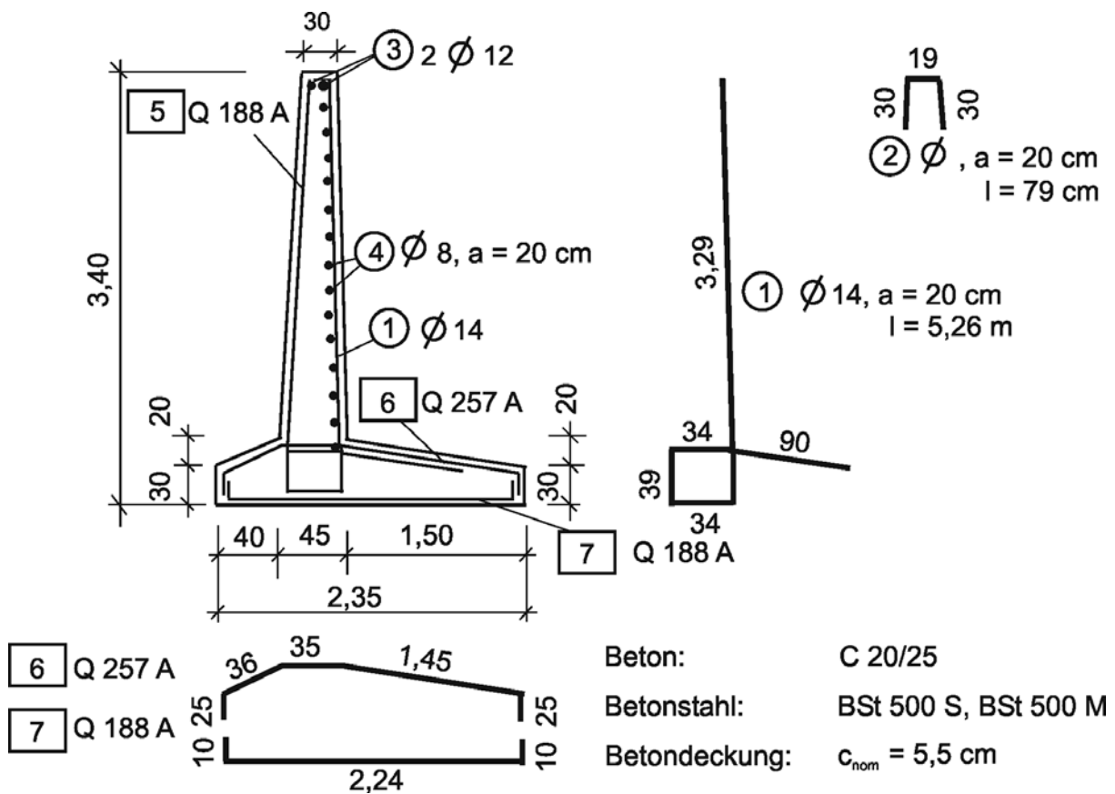
6-26 Bewehrung einer Winkelstützmauer
