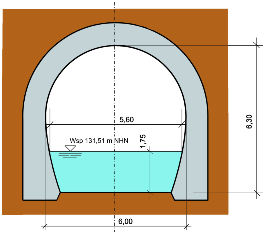
16-25 Schiffahrtstunnel bei Weilburg/Lahn
