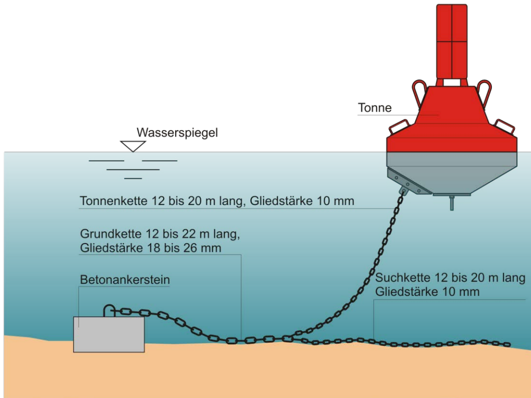
13-5 Tonneverankerung auf kiesiger Flusssohle
