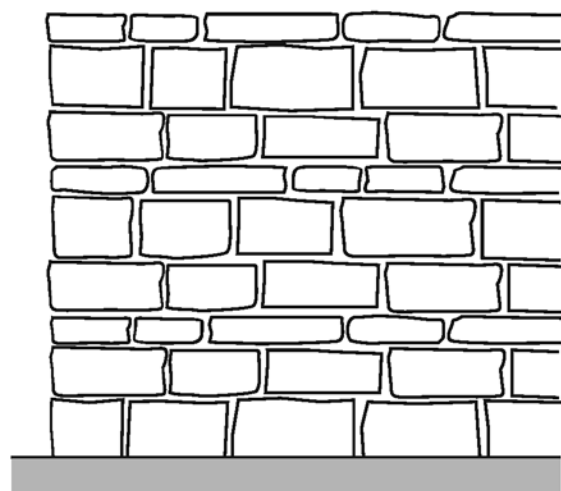
Regelmäßiges Schichtenmauerwerk
