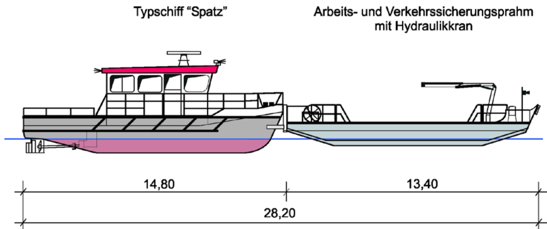
14-1 Typsystem „Spatz“
