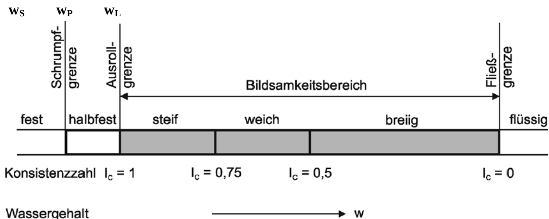
6-32 Konsistenzbalken nach Atterberg
