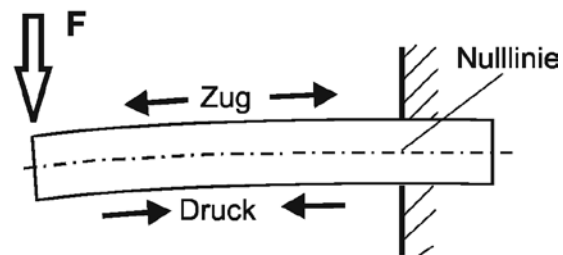
6-23 Kragträger
