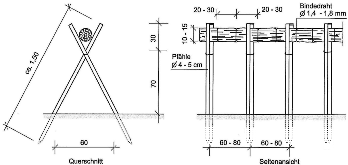
15-10 Wippe mit Wurstbank
