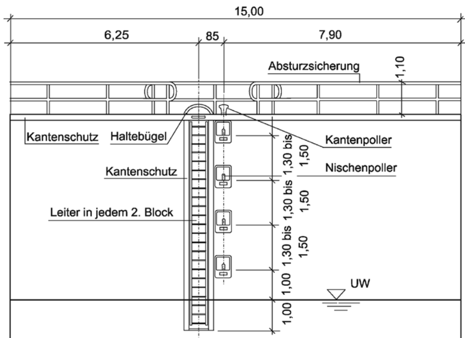
16-17 Regelblock einer Schleusenammer
