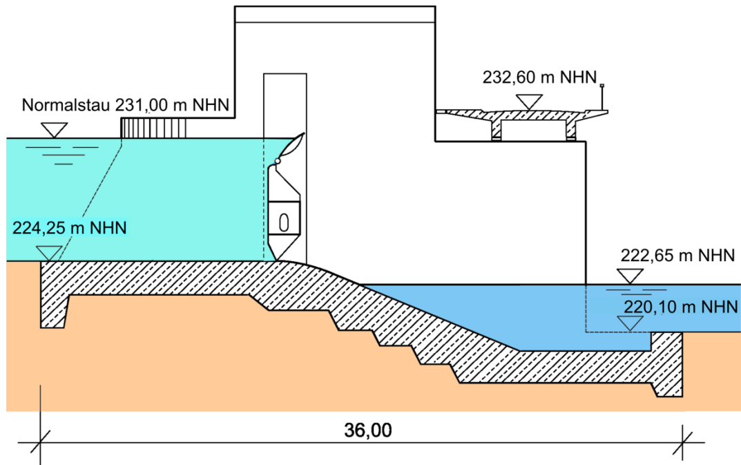
16-6 Wehr mit Rollenschütz und Aufsatzklappe in Obertürkheim/Neckar (Inbetriebnahme 1968)
