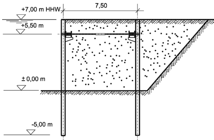
15-35 Querschnitt eines Kastenfangedammes
