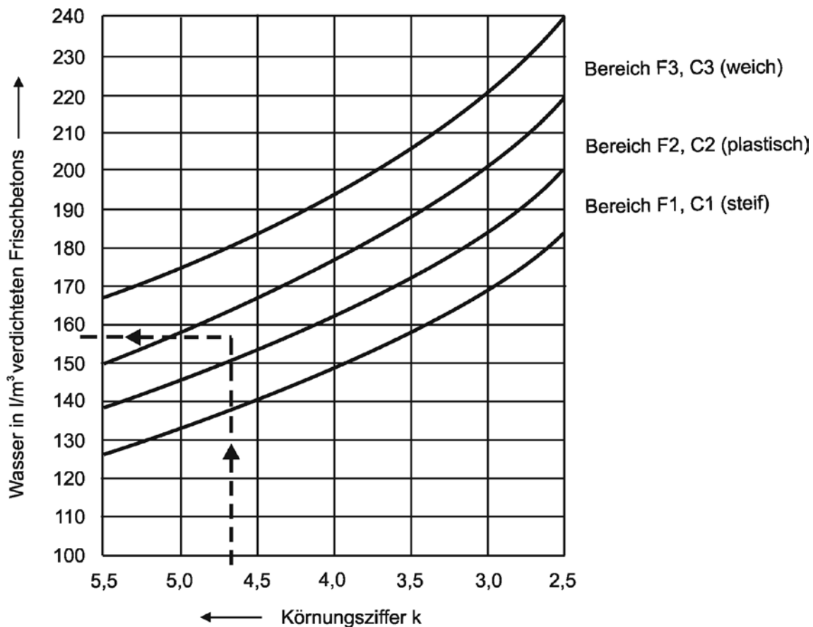
6-11 Wasseranspruch des Betons (nach Schwenk „Betontechnische Daten“)
