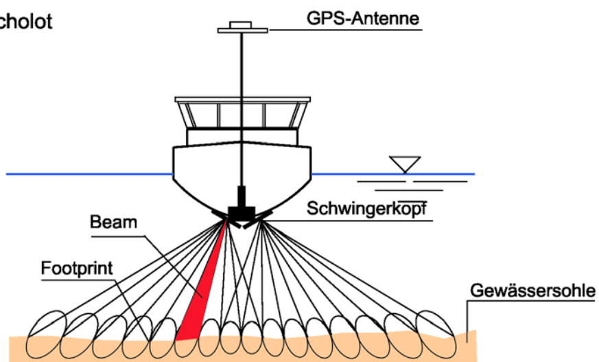
9-6 Messsysteme für die Tiefenmessung
