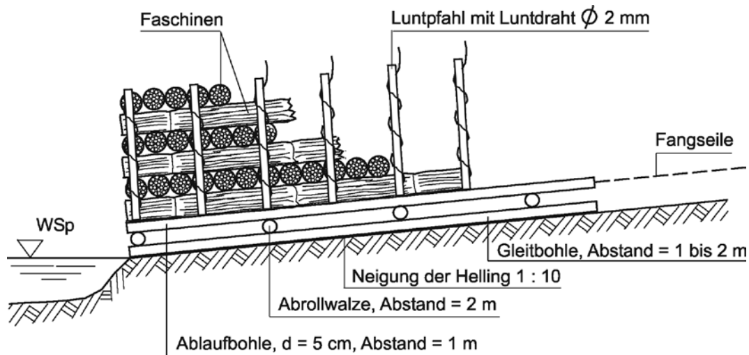
15-19 Sinkstück auf der Helling (Querschnitt)
