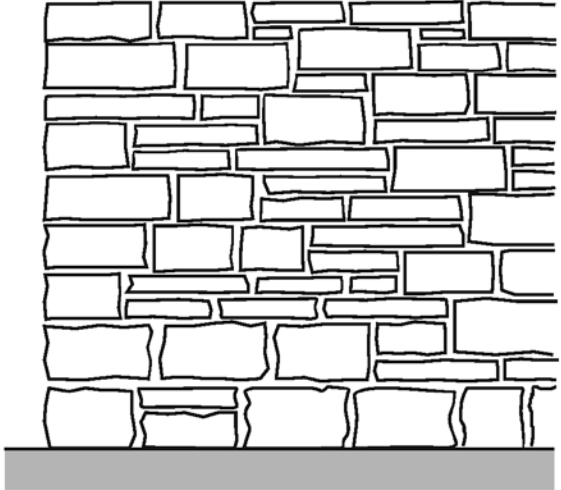
Hammerrechtes Schichtenmauerwerk
