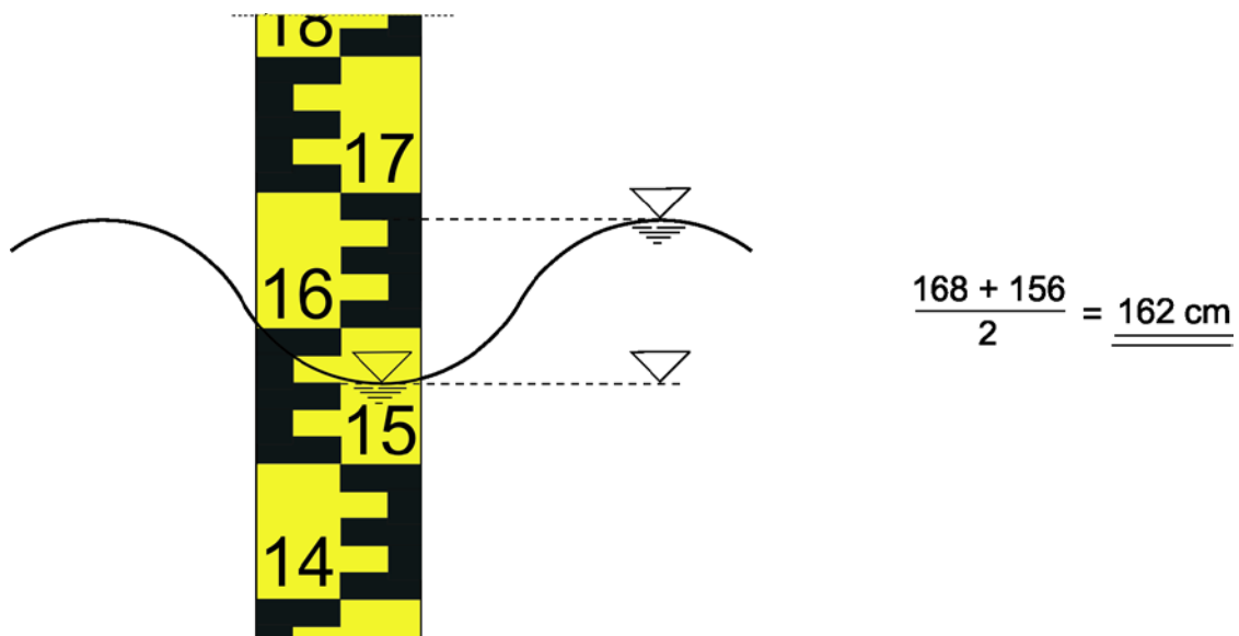
10-5 Ablesung bei unruhigem Wasserstand
