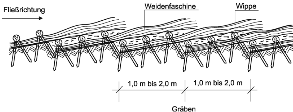
15-18 Rauwehr (Längsschnitt durch die Böschung)
