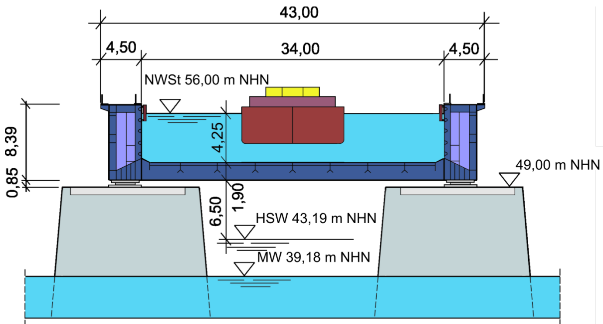
16-24 Querschnitt der Kanalbrücke Magdeburg im Strombereich
