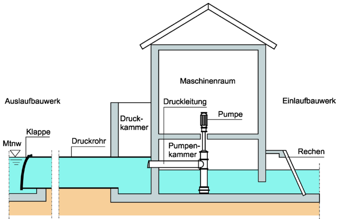
19-8 Schematischer Schnitt eines Schöpfwerkes
