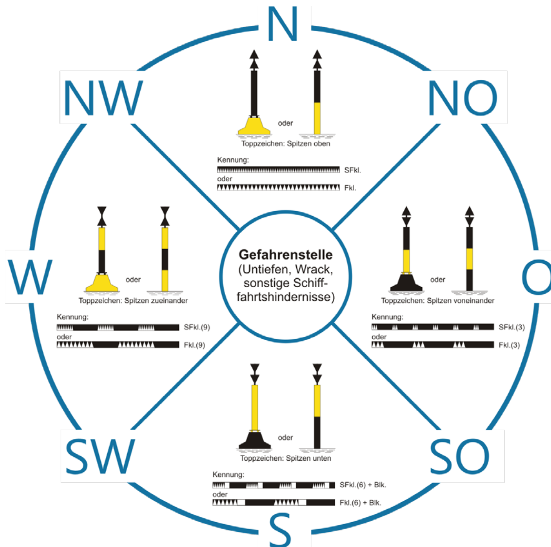
13-40 Bezeichnung von Gefahrenstellen
