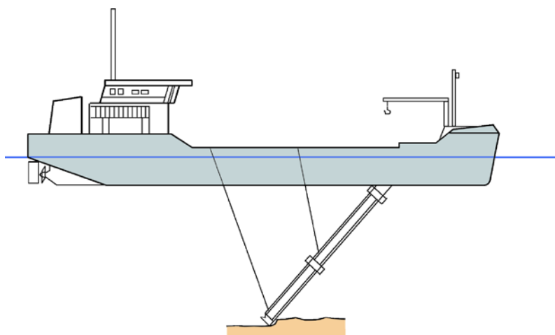
14-5 Hopperbagger (Laderaumsaugbagger)
