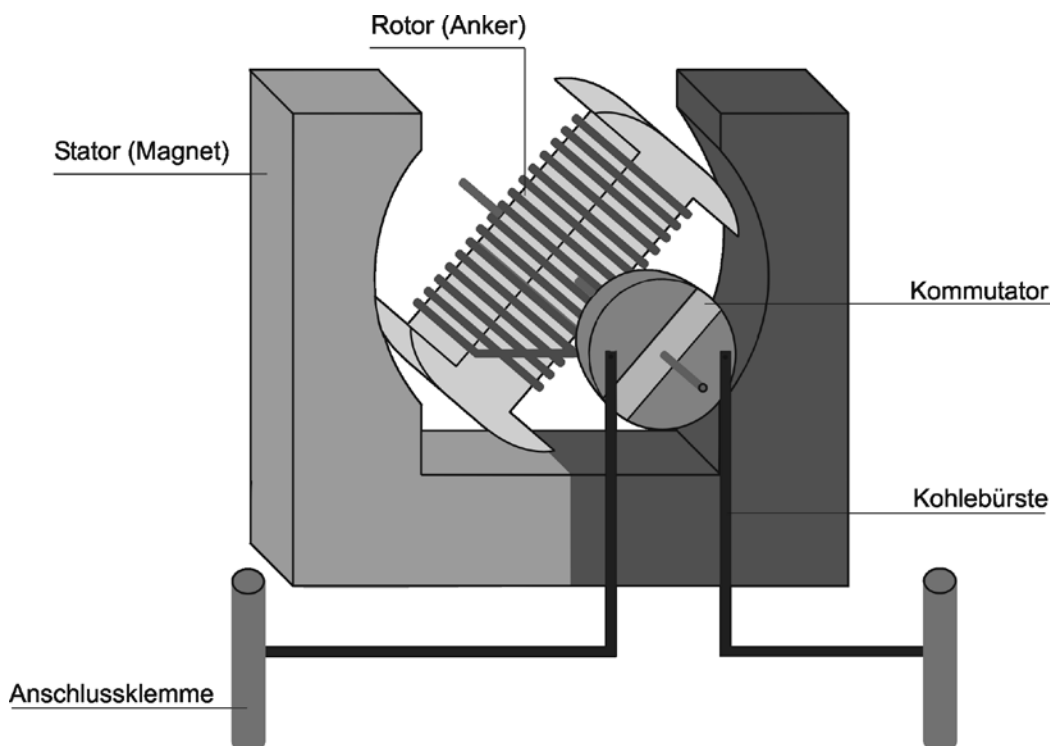
7-1 Prinzip des Elektromotors
