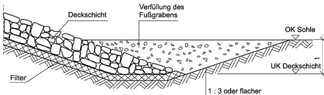
15-28 Fußeinbindung (Fußverlängerung)
