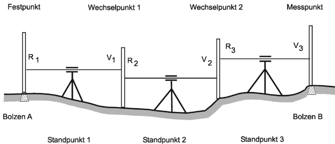
8-8 Liniennivellement
