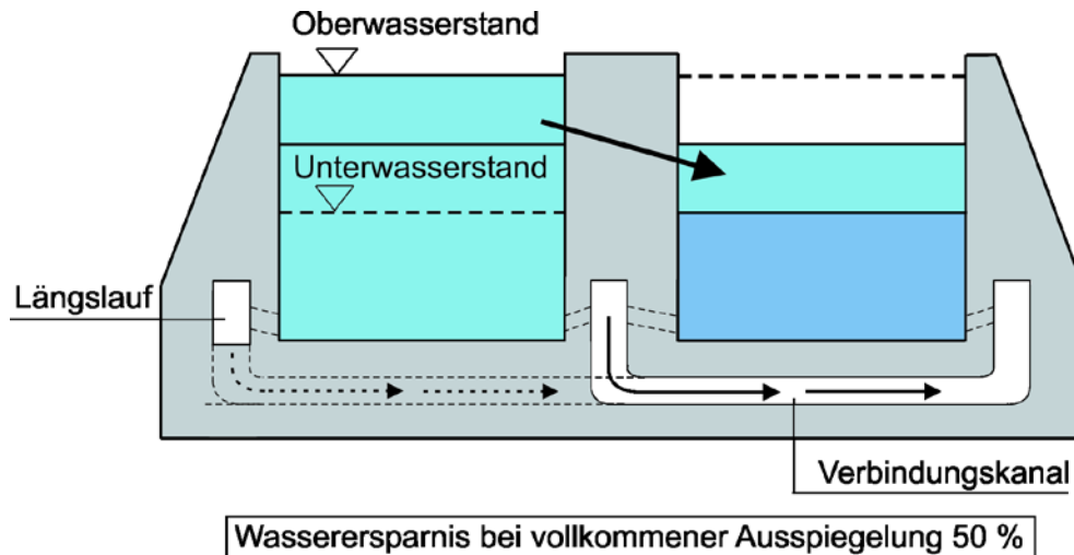
16-13 Zwillingsschleuse
