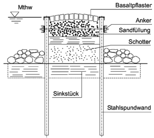
19-14 Kastenbuhne (Querschnitt)
