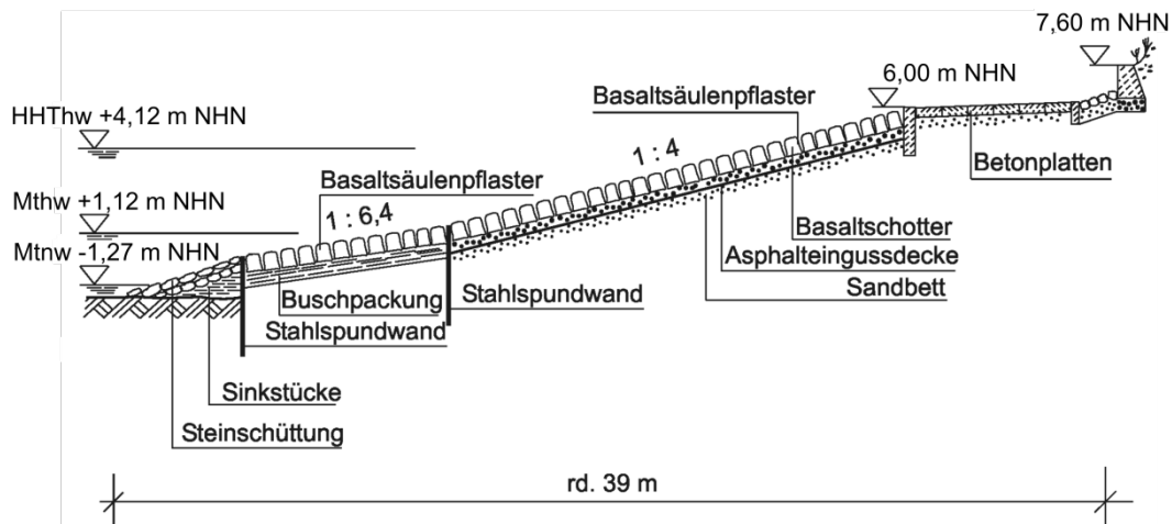
19-11 Schrägdeckwerk auf Norderney (nach Unterlagen des Niedersächsischen Landesbetriebes für Wasserwirtschaft, Küsten- und Naturschutz (NLWKN))
