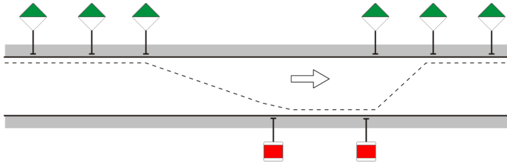
13-29 Zusammenspiel der Bilder 13-25 und 13-27
