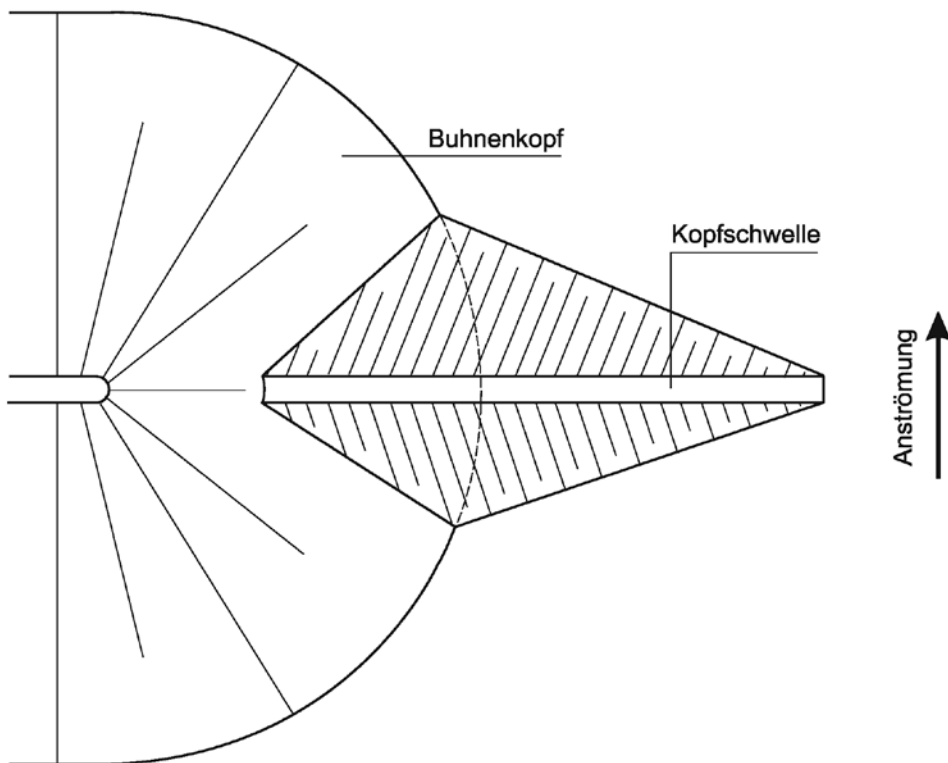
12-12 Kopfschwelle
