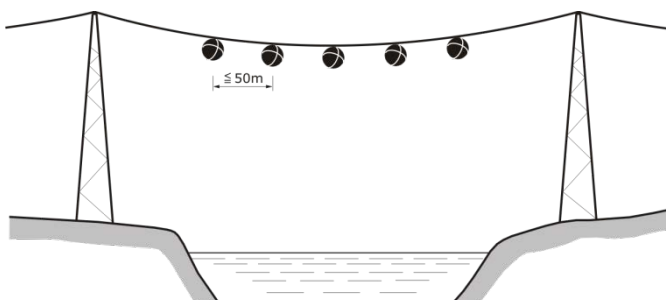
13-23 Radarreflektoren an Freileitung
