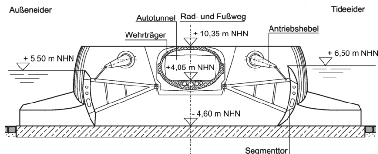
19-6 Eidersperrwerk (Querschnitt)
