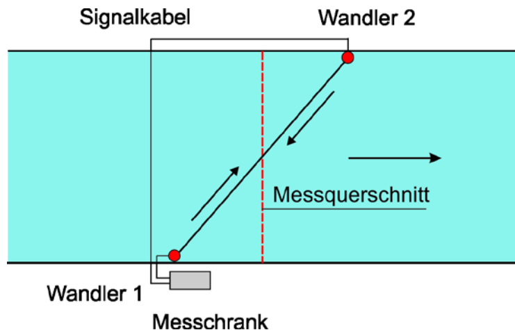
10-20 Ultraschall-Laufzeitanlage
