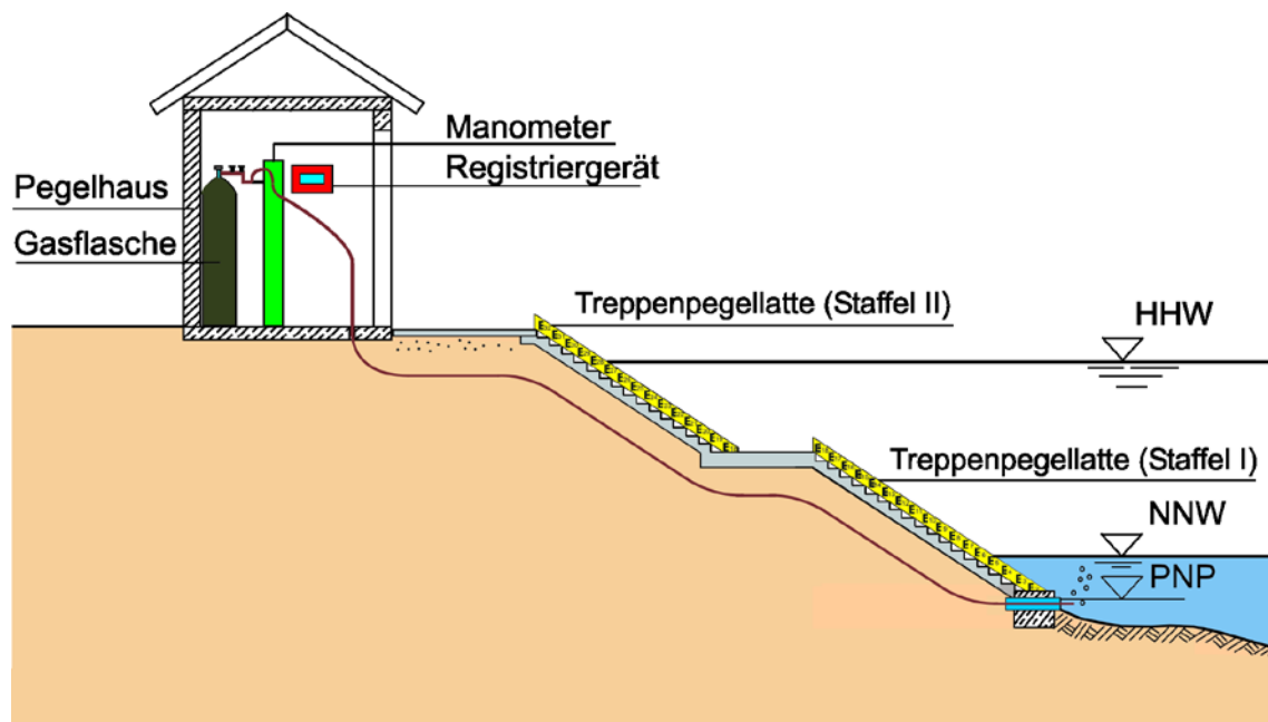
10-10 Druckluftpegel (Einperlmethode)
