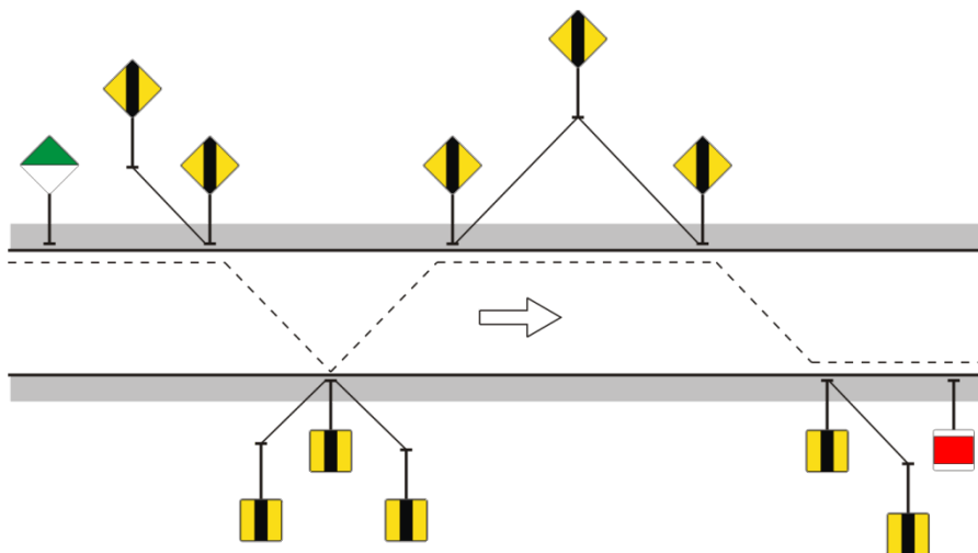
13-35 Bezeichnung durch Richtbaken
