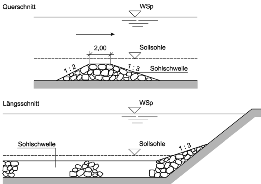
12-14 Sohlschwelle
