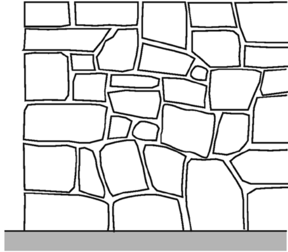
Zyklopenmauerwerk
