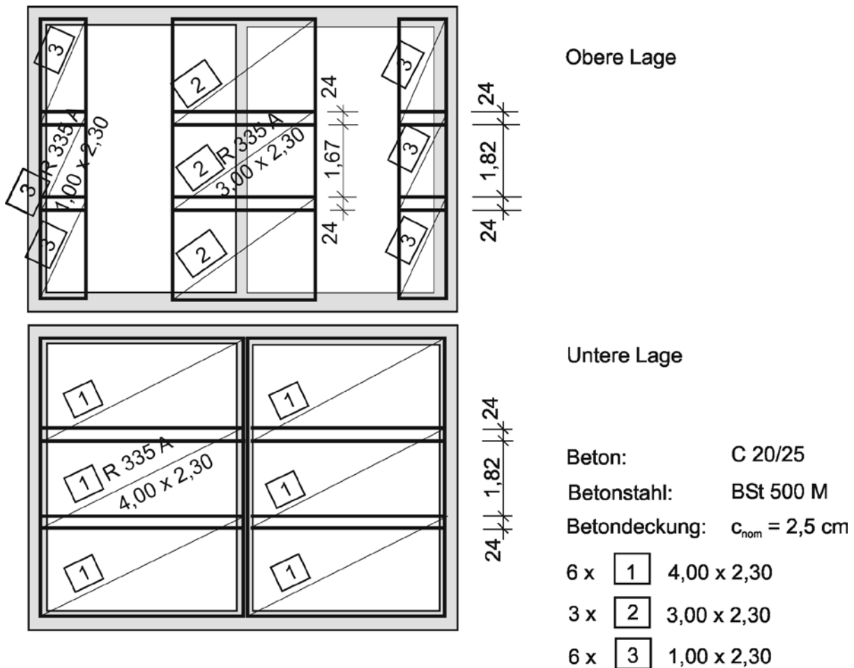
6-27 Deckenbewehrung
