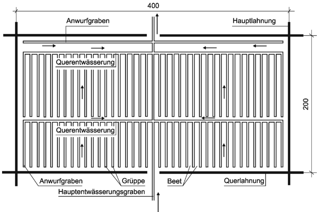
19-17 Lahnungsfeld
