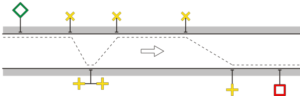
13-34 Bezeichnung durch Einzelbaken
