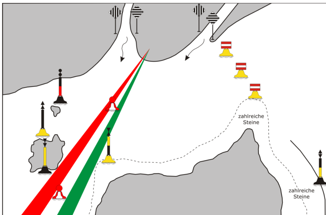
13-46 Zusammenspiel der Bilder 13-36 bis 13-45 und Bild 13-48
