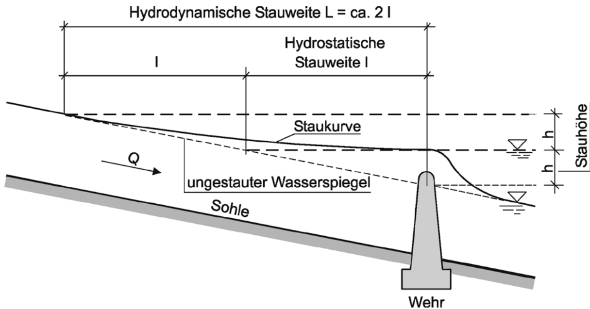
12-15 Staubereich einer Stauhaltung
