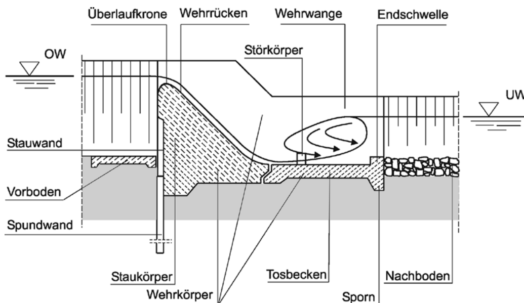
16-1 Bestandteile des festen Wehres
