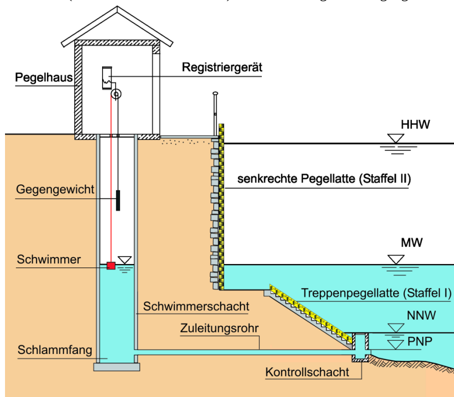
10-9 Mechanischer Schwimmerschreibpegel
