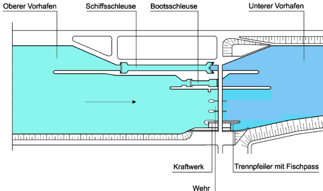
12-16 Bauwerke einer Staustufe
