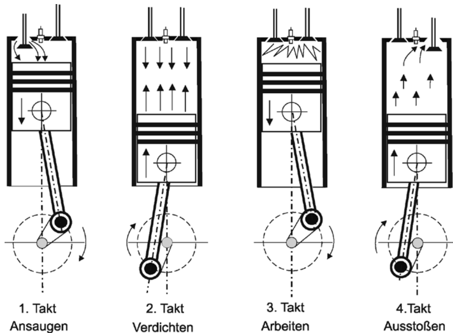
7-3 Viertakt-Arbeitsverfahren
