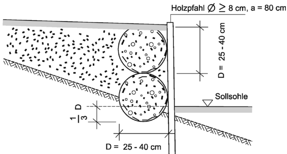
15-11 Faschinenwalzen
