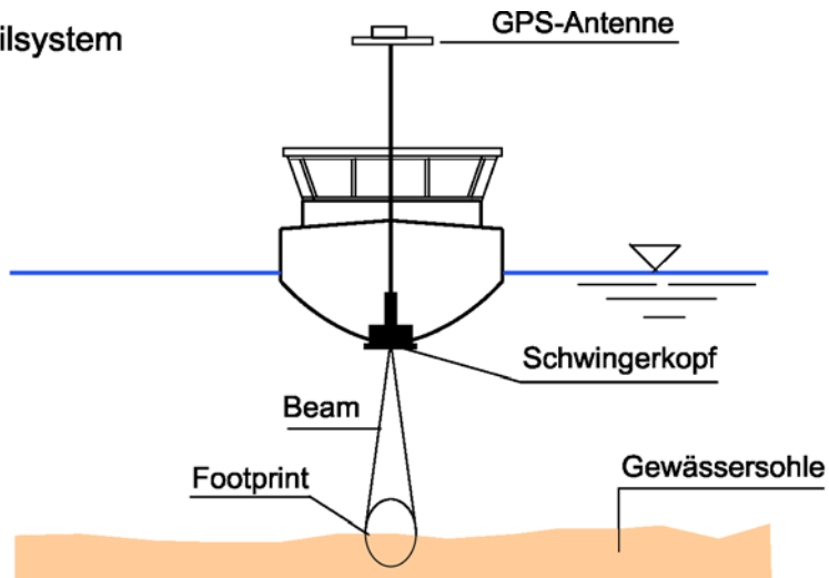
Auslegersystem
