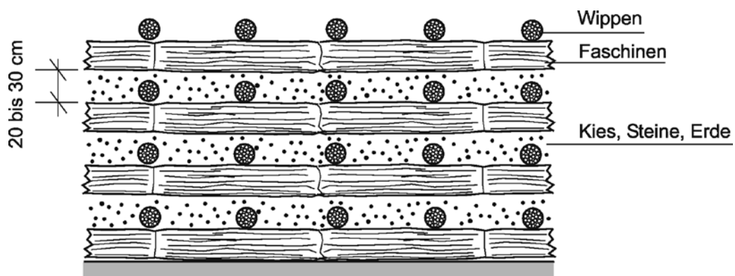
15-16 Packfaschinat
