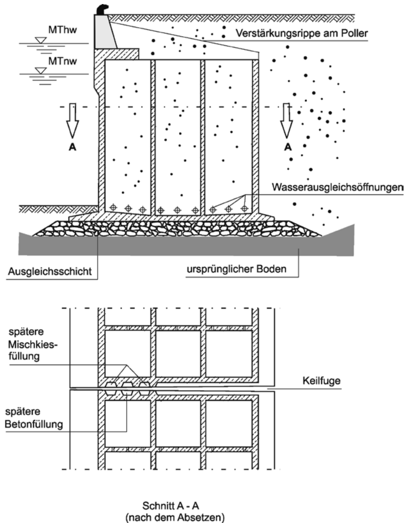
15-41 Ufermauer aus Schwimmkästen (EAU 2004)
