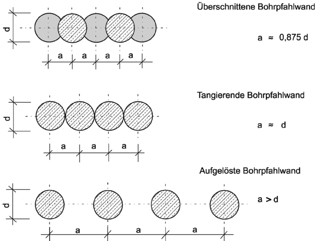
15-36 Bohrpfahlwände (Empfehlungen des Arbeitsausschusses Ufereinfassungen (EAU 2004))
