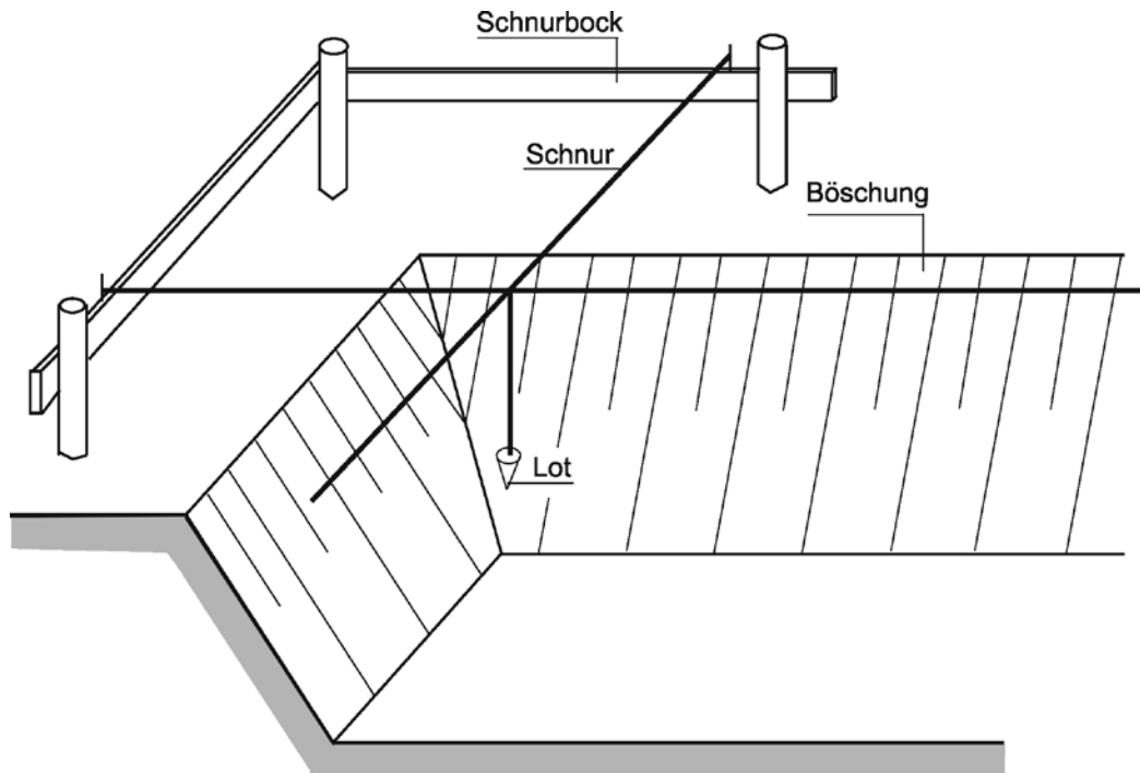
8-3 Baugrube mit Schnurgerüst
