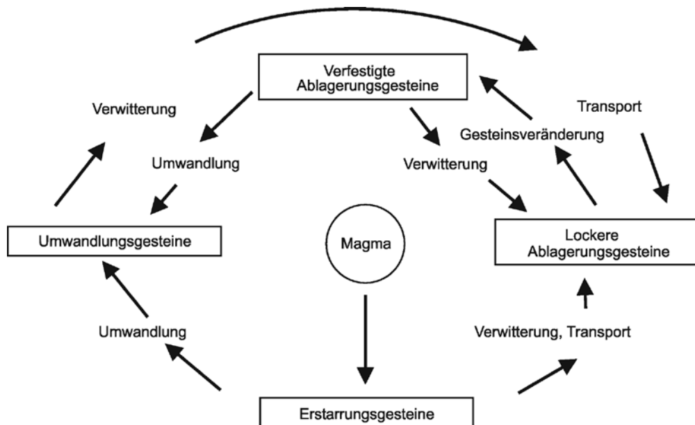
6-3 Kreislauf der Gesteine (nach W. Schumann „Steine und Mineralien“)
