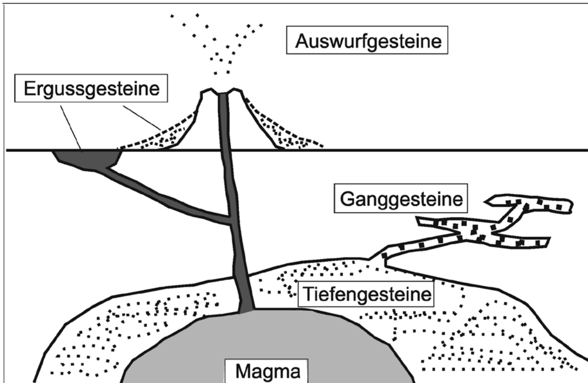
6-5 Entstehung der Erstarrungsgesteine (nach W. Schumann „Steine und Mineralien“)
