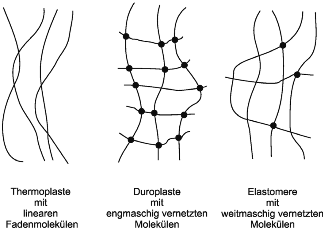
6-37 Aufbau der Makromoleküle
