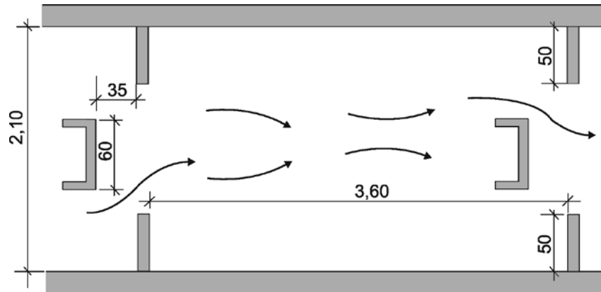
16-27 Schlitzpass der Staustufe Bremen (Draufsicht)
