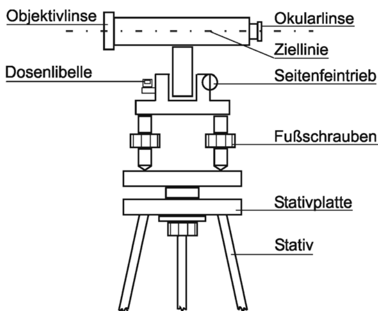
8-1 Automatisches Nivelliergerät
