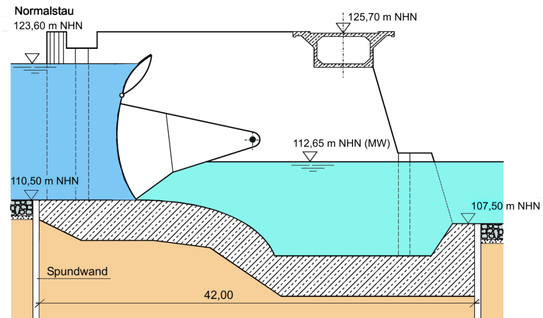
16-7 Drucksegmentwehr mit Aufsatzklappe in Iffezheim/Rhein (Inbetriebnahme 1977)
