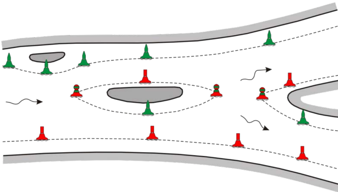
13-10 Bezeichnung der Fahrrinne durch schwimmende Zeichen
