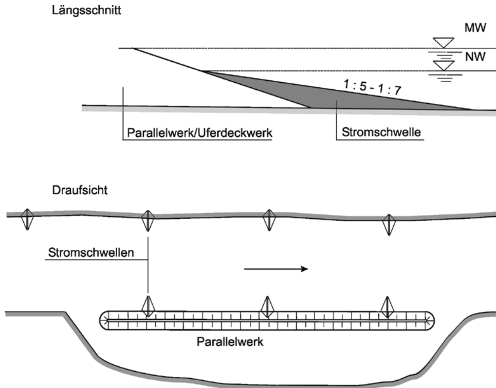
12-13 Stromschwellen
