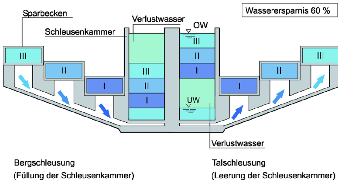
16-14 Schematischer Querschnitt einer Doppelschleuse mit Sparbecken
