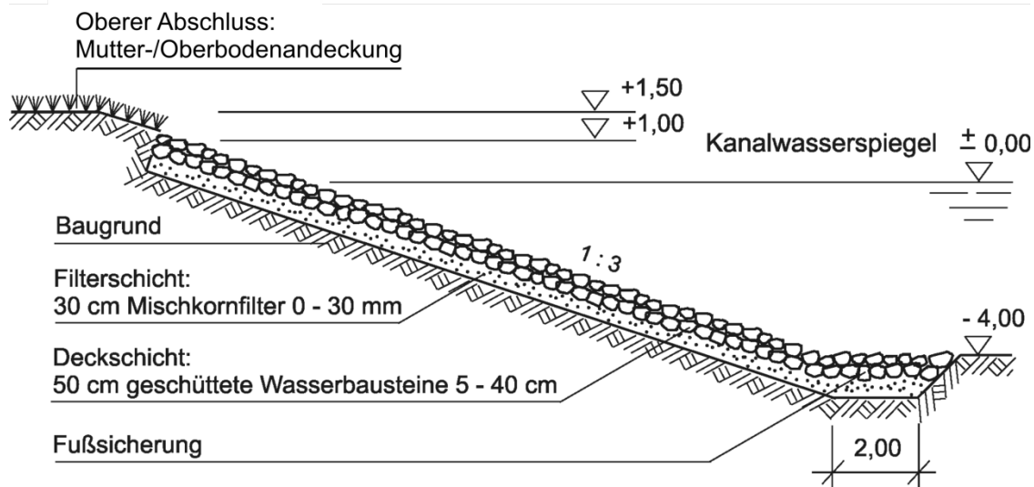
15-20 Durchlässiges Uferdeckwerk
